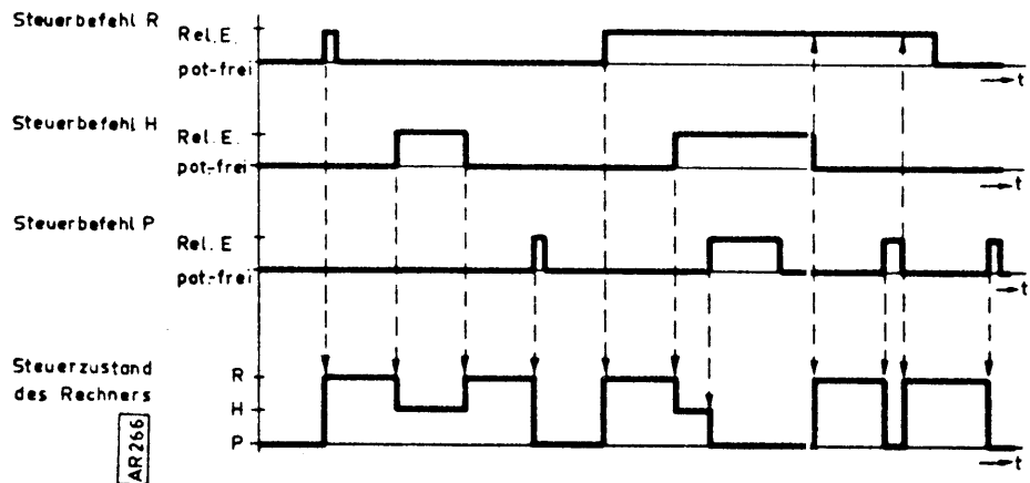
Bild 5: Externe Steuerbefehlsfolge
