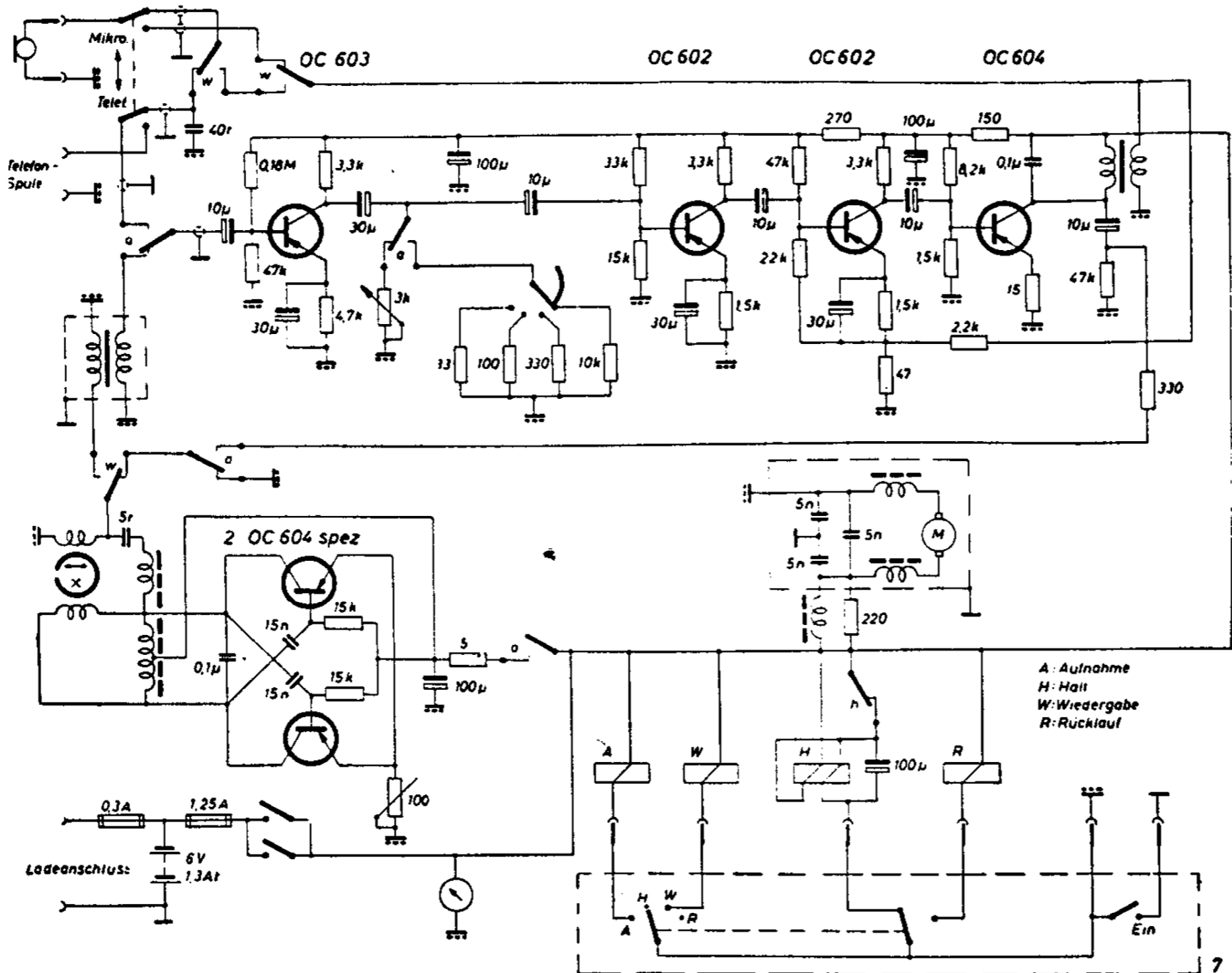
Lo schema del Traveller; sotto, lo schema della testina.
