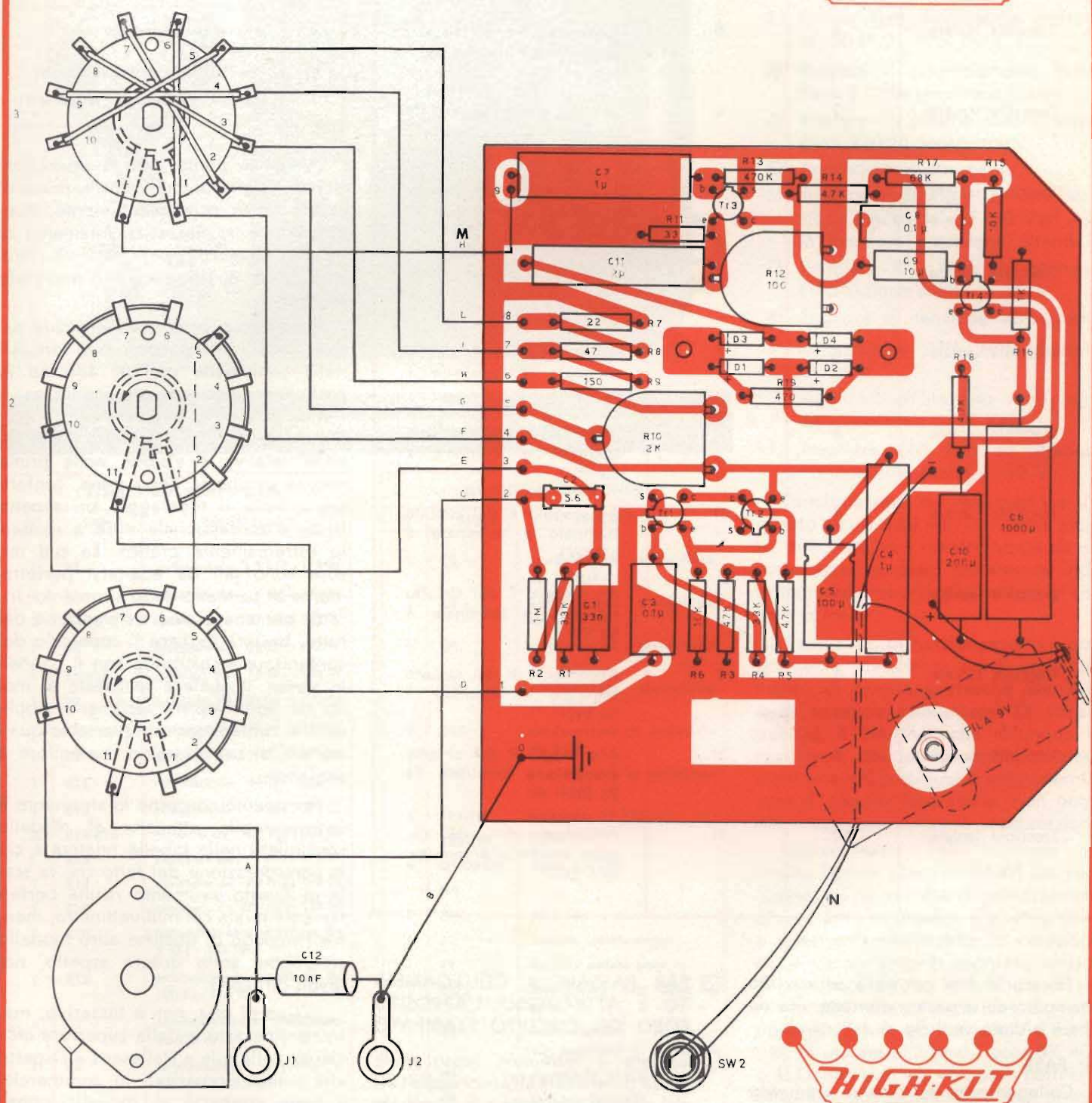
Fig. 6 - Cablaggio completo dello strumento.
