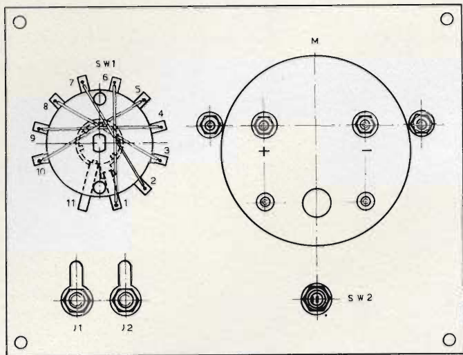
Fig. 4 - Montaggio delle parti staccate sul pannello frontale.
