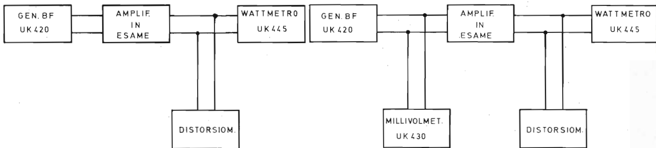
Fig. 6 - Schema a blocchi del circuito di misura per il rilievo della curva della potenza in funzione del carico.
