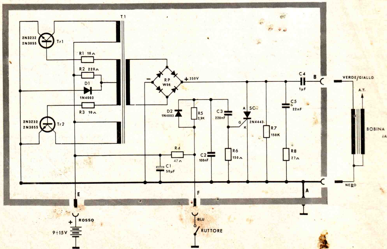
Fig. 4 - Circuito elettrico dell'accensione elettronica transistorizzata UK875.
