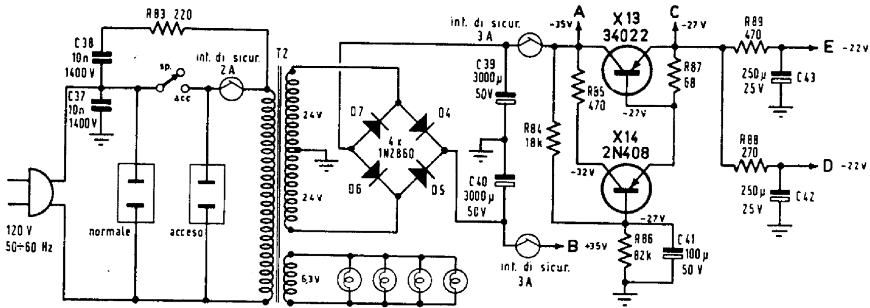
- Schema elettrico dell'alimentatore.
