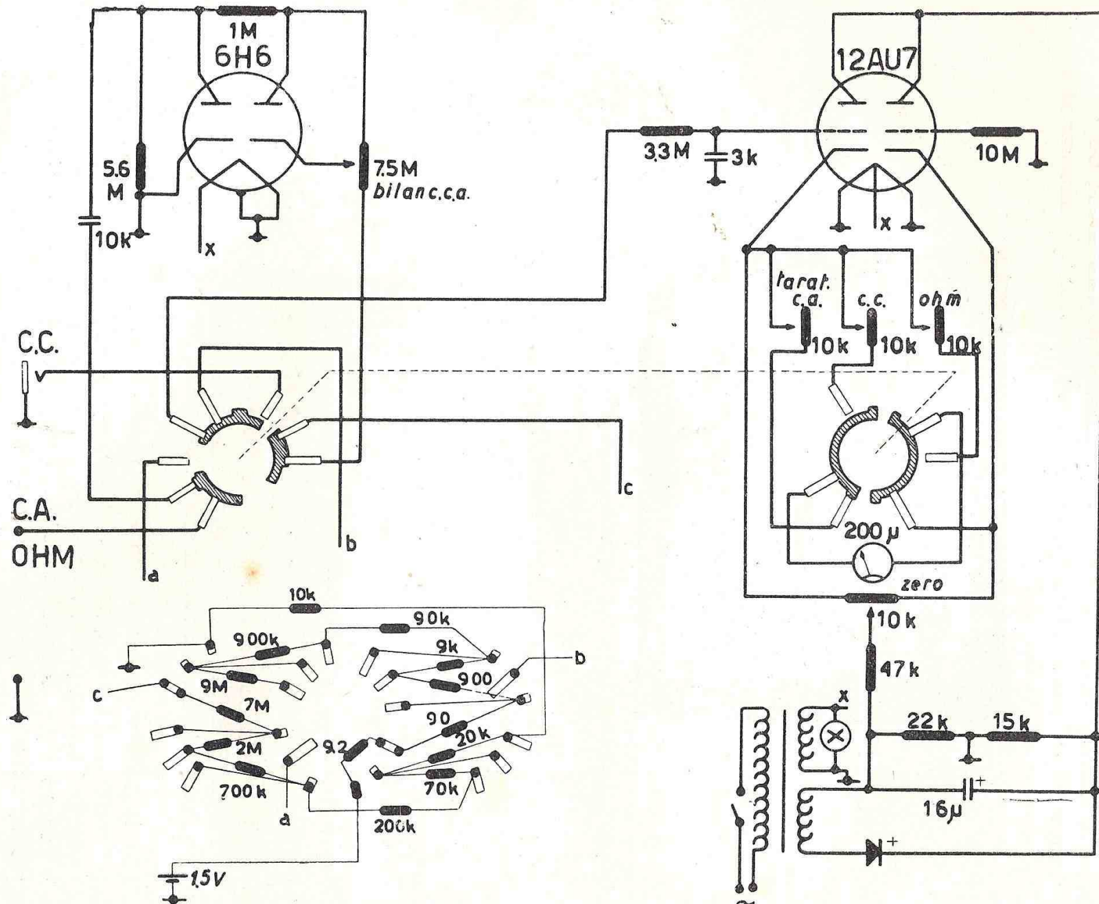
Fig. 65. - Voltmetro elettronico Heath V-6.
