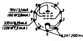
EF 89
