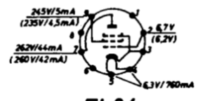
EL 84
