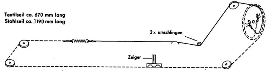
FM-Antrieb von der Skalenseite gesehen
