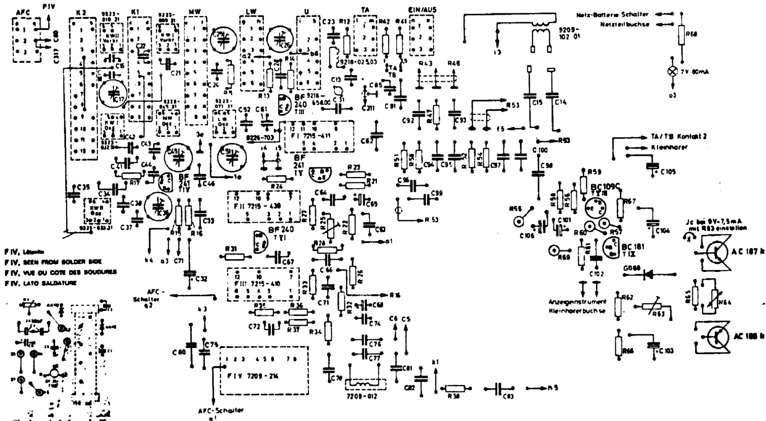
PIASTRA CIRCUITI STAMPATI, LATO SALDATURE
