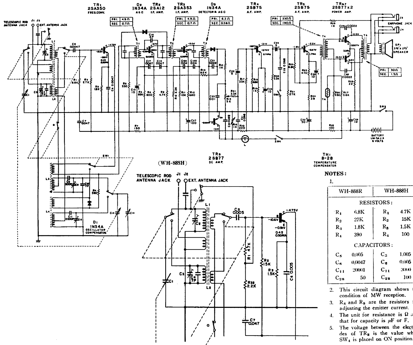
Schema elettrico del radiorecettore a transistor HITACHI mod. WH 888 R WH 888 H
