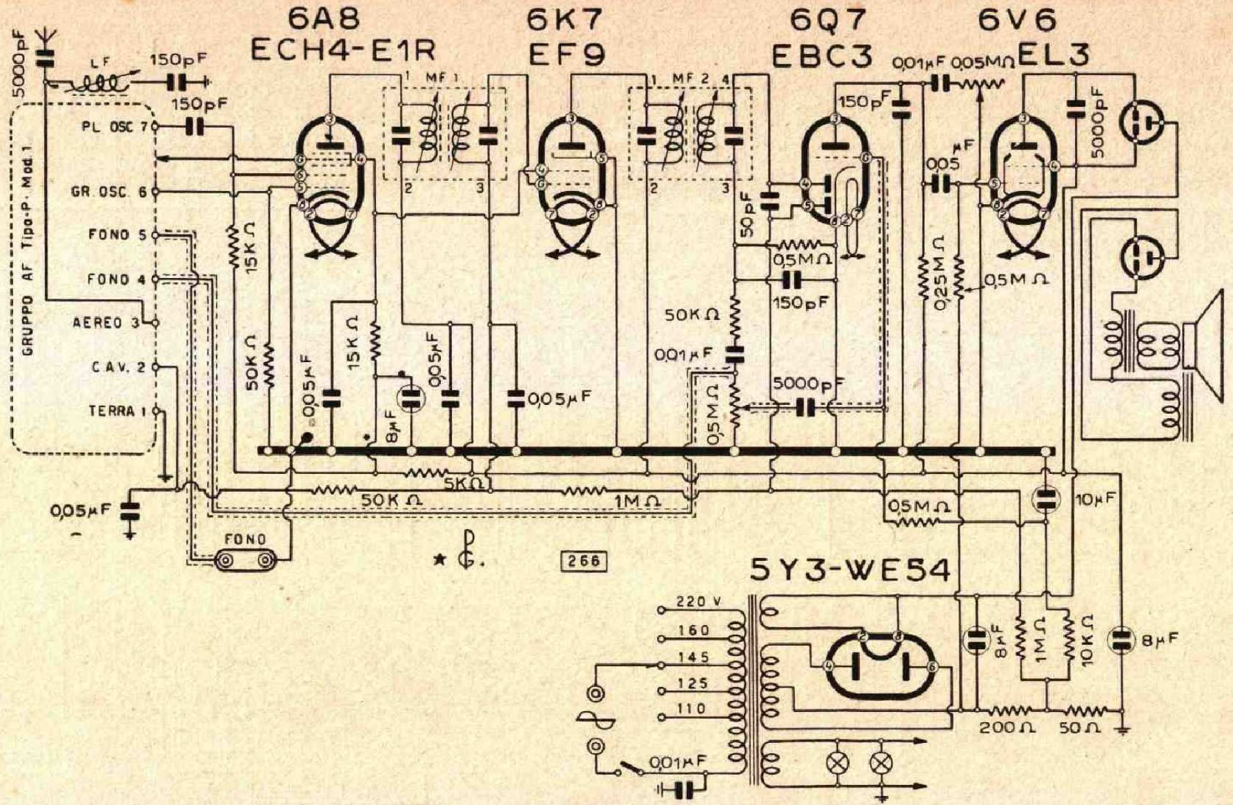
Lo schema elettrico del mod. 503 (5A5) (SC4)
