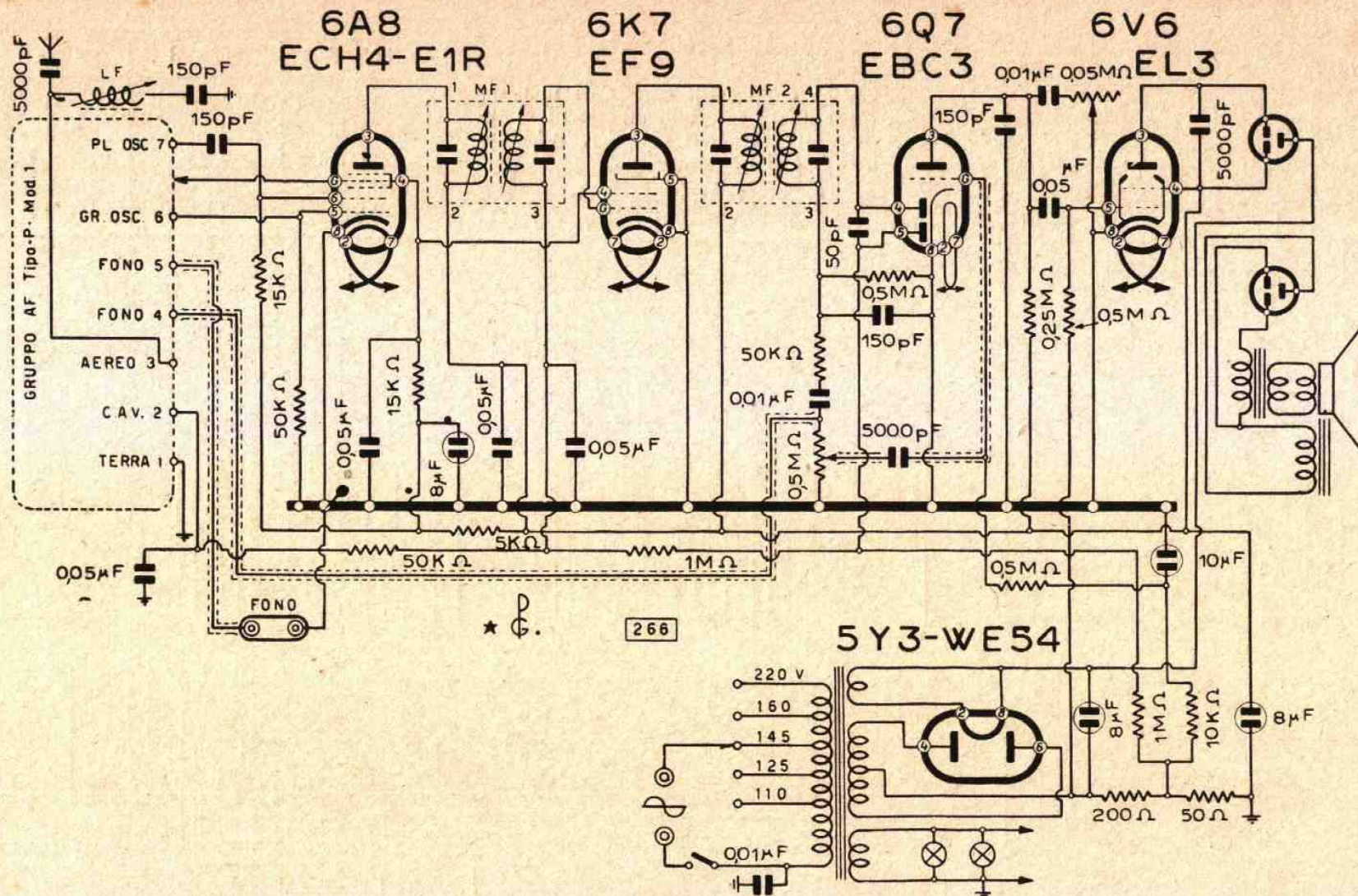
Lo schema elettrico del mod. 503 (5A5) (SC4)
