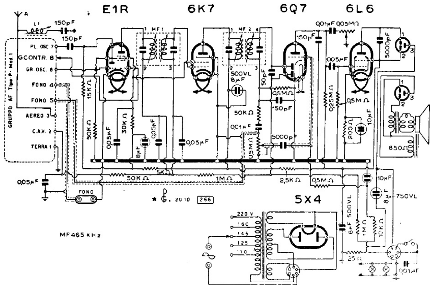
Lo schema elettrico del mod. 505 (SC4).
