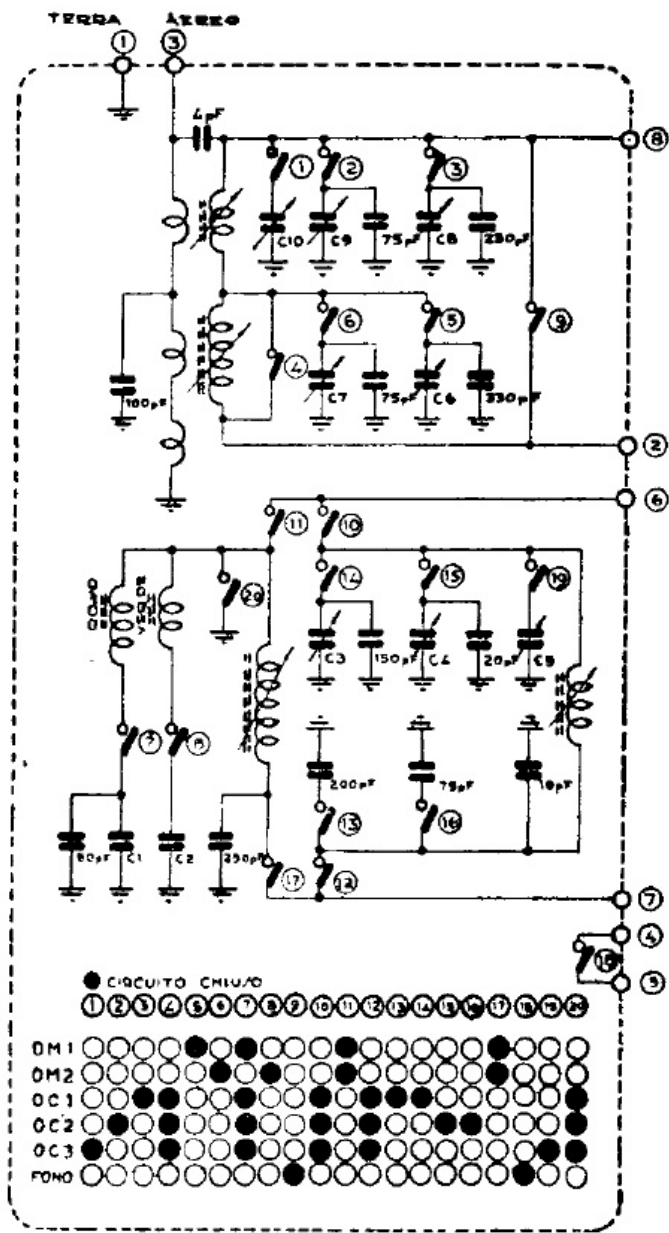
Il gruppo AF Nova P1 impiegato nei ricevitori descritti in questa scheda.
