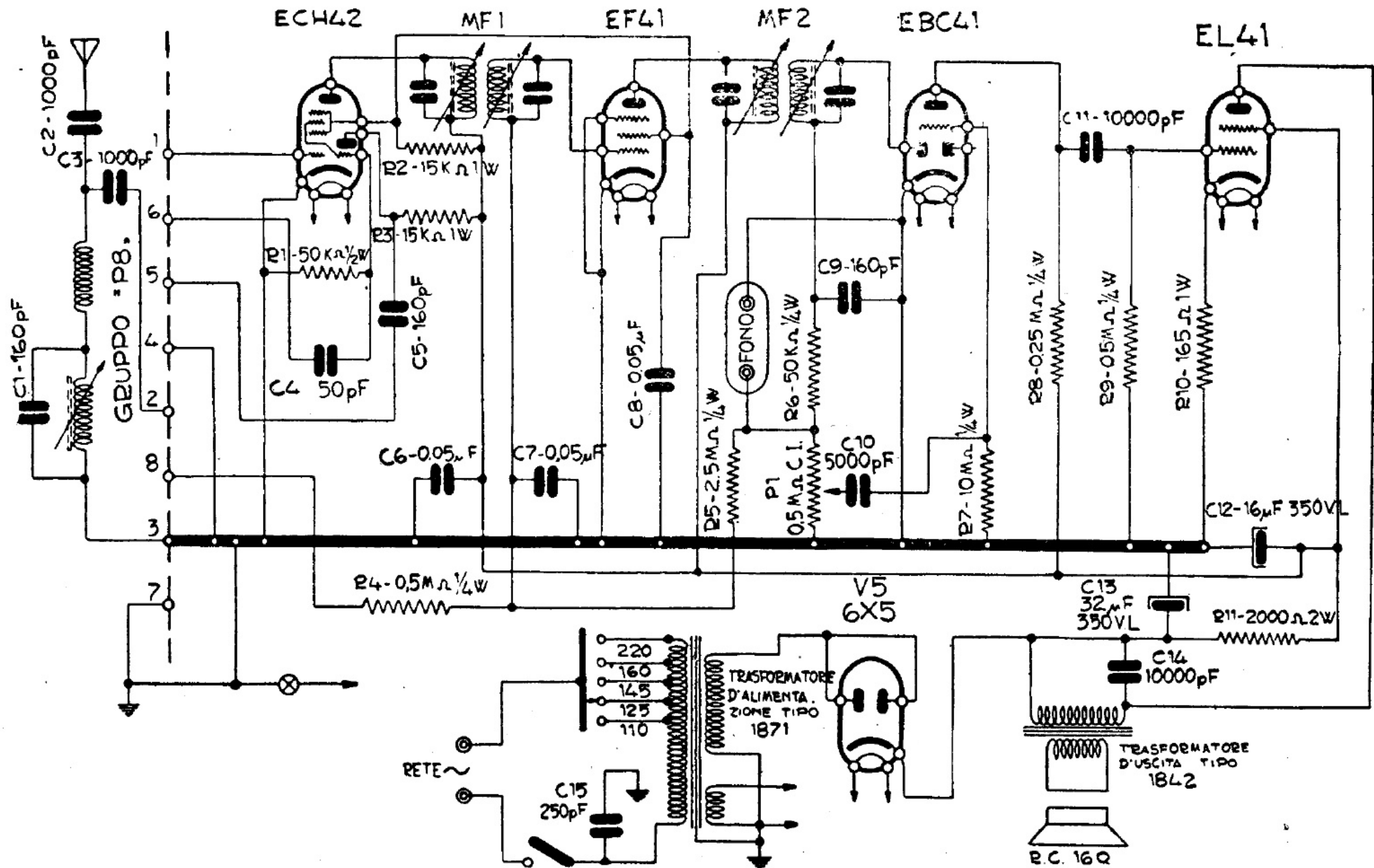
NOVA RADIO - Mod. A.2 - Medie divise, corte divise. Media frequenza 465 kc. Finale: 205 V placca, 175 V schermo, 4,2 V catodo. Uscita: 4 W su 5 ohm.
