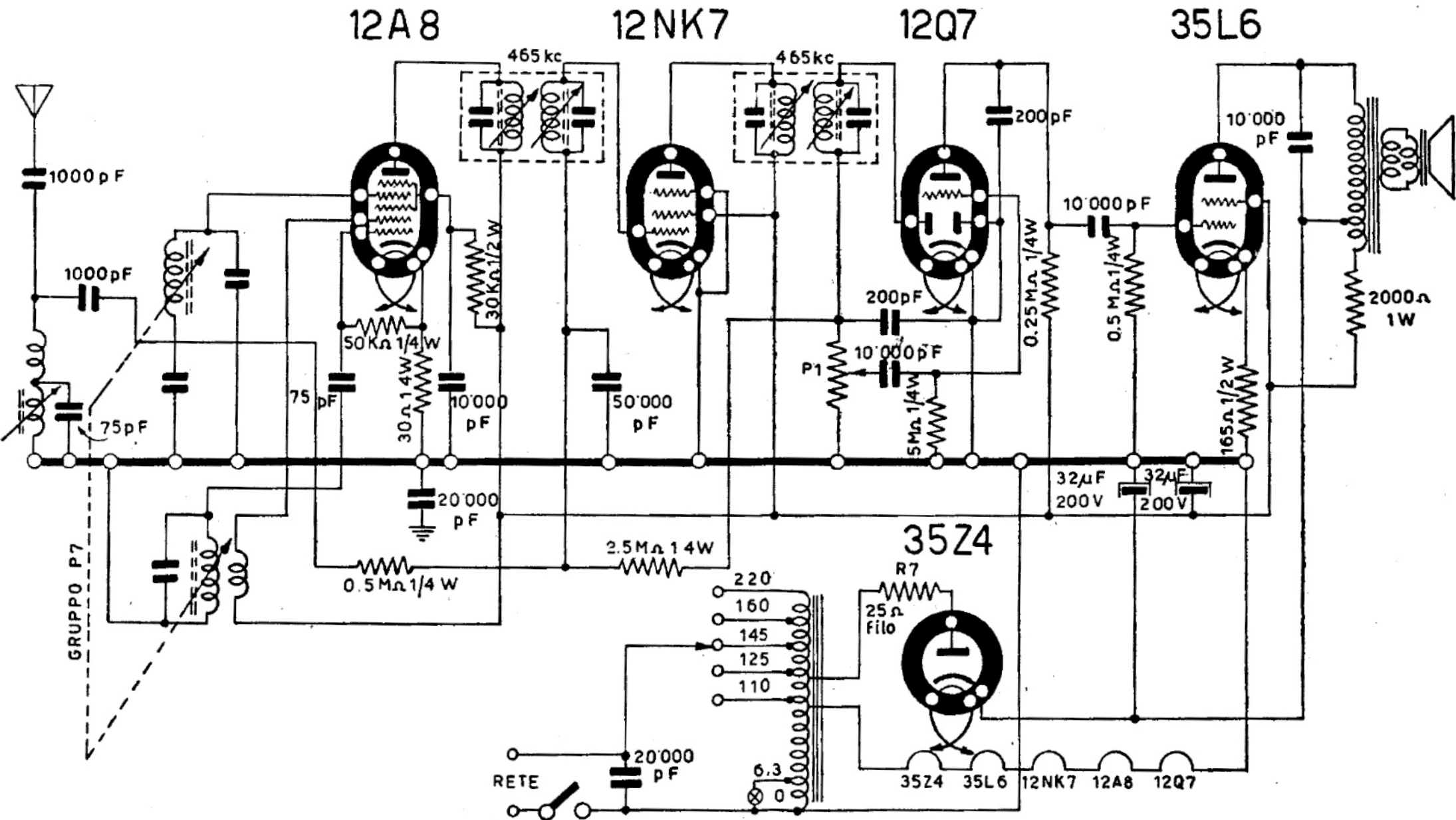
NOVA RADIO - Modd. AR48, 5L1 e 5L2 (Chassis 512) - Gamma medie da 517 a 1620 kc/s. Media frequenza 465 kc/s. Potenza d'uscita 2 W. (Il mod. 5L2 è identico salvo il gruppo AF che è il P8 a due gamme d'onda).
