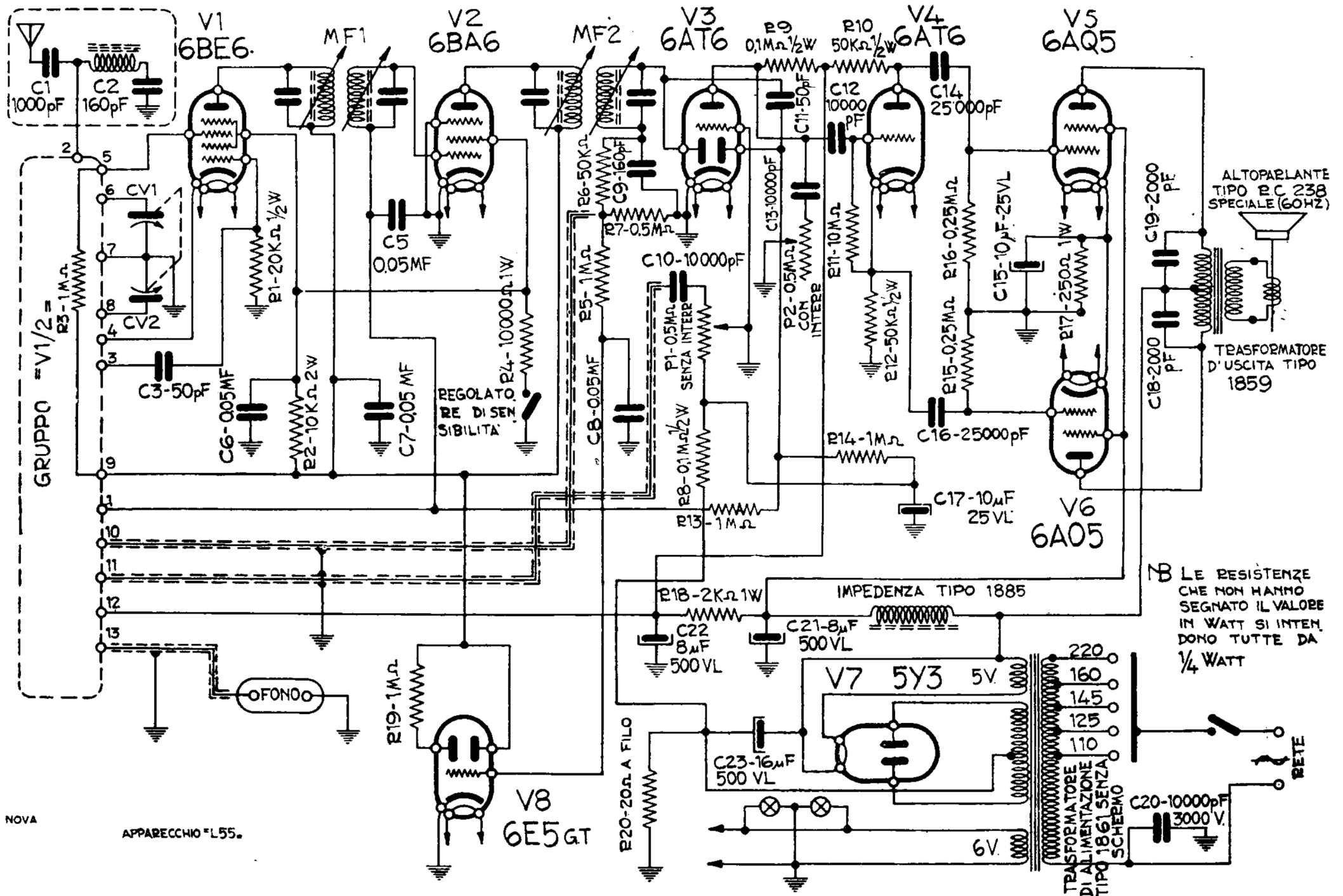
NOVA - Mod. L55. Ricevitore con sintonia a permeabilità variabile, provvisto di gruppo AF mod. V1/2. Media frequenza 465 kc/s. Potenza indistorta di uscita 8 watt. Consumo 60 watt.
