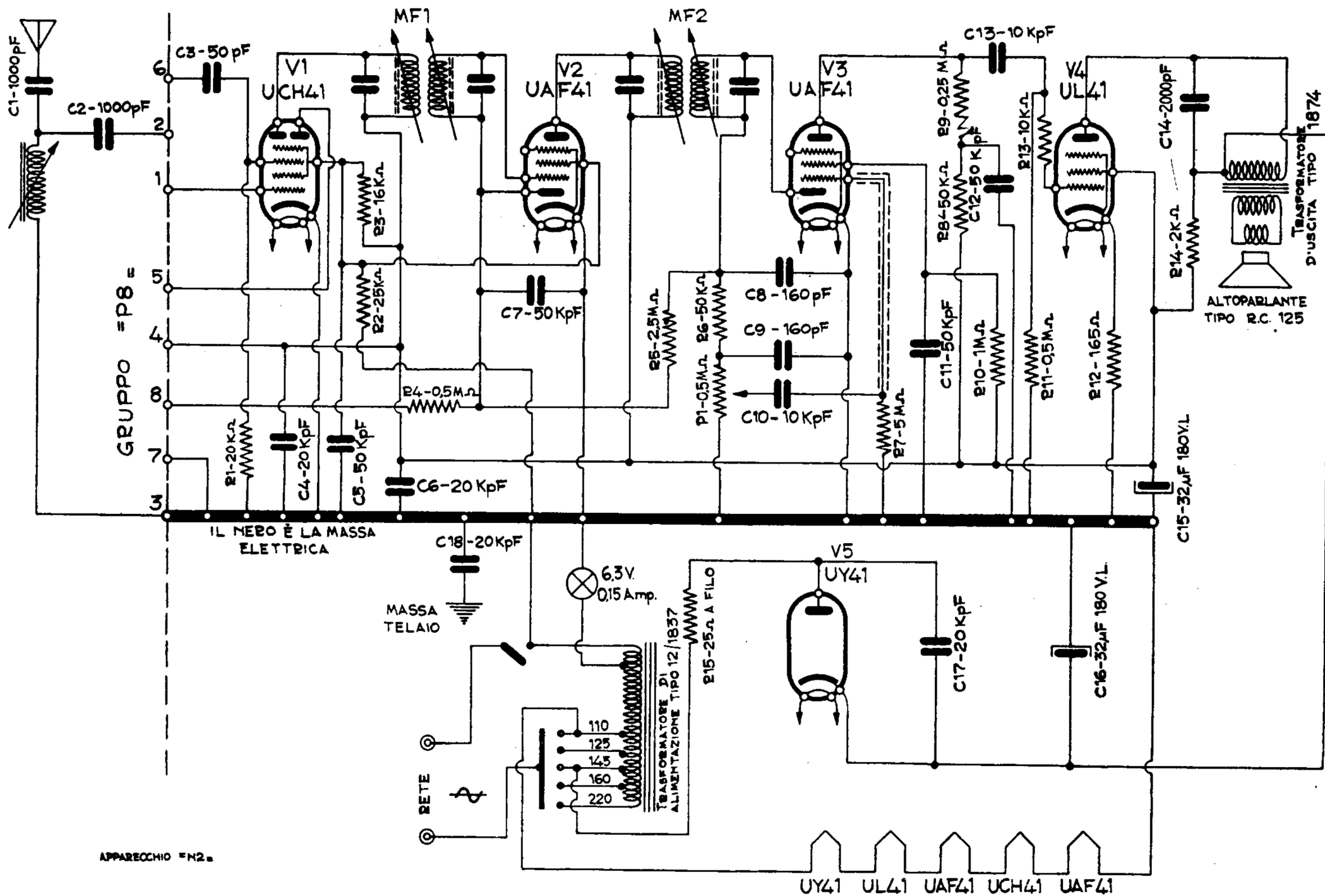
NOVA - Mod. N2. Ricevitore con sintonia a permeabilità variabile, provvisto di gruppo AM mod. P8. Media frequenza 465 kc/s. Resa di uscita 2 watt. Consumo 35 watt.
