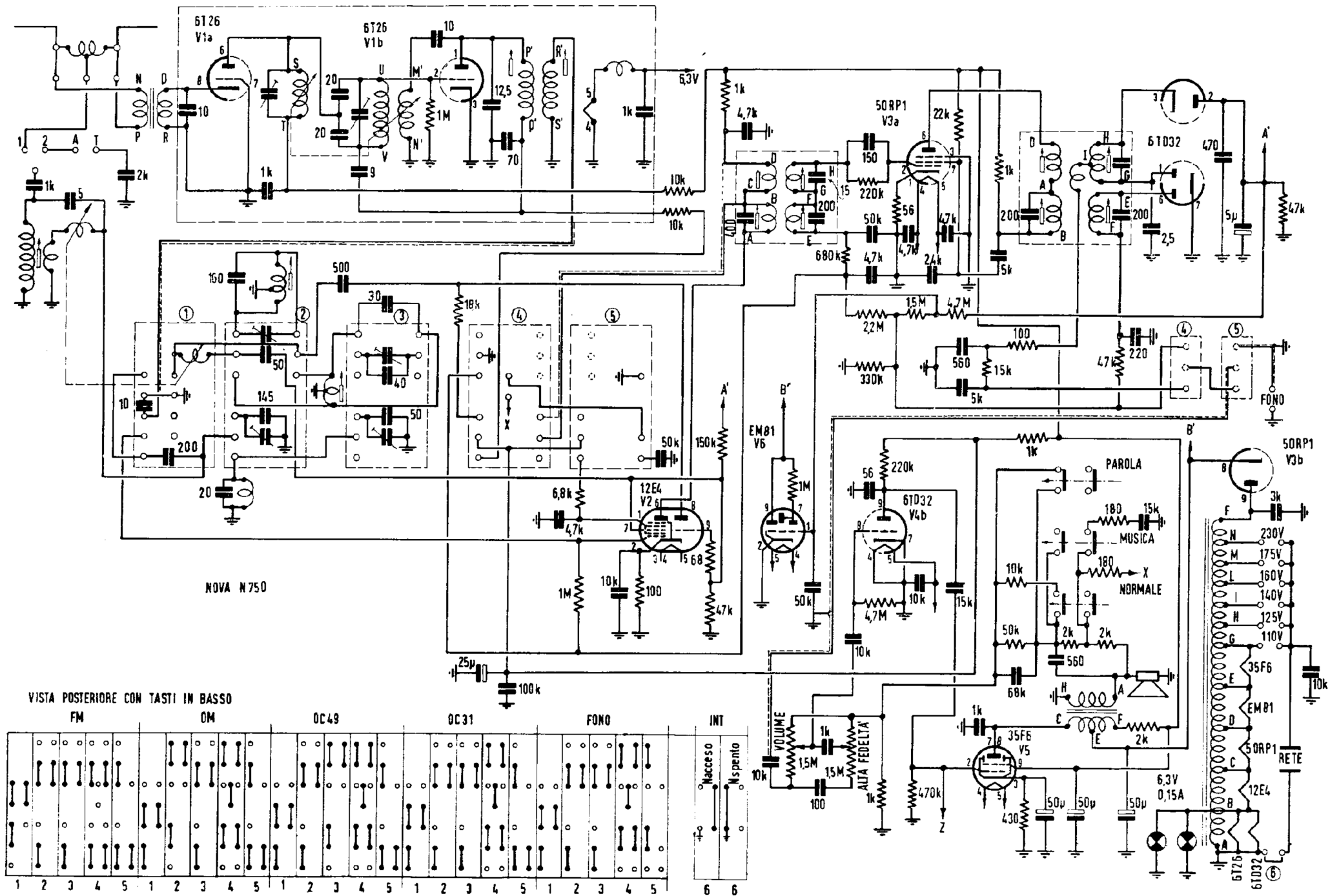
Schema elettrico del radiorecettore AM-FM, Nova N 750
