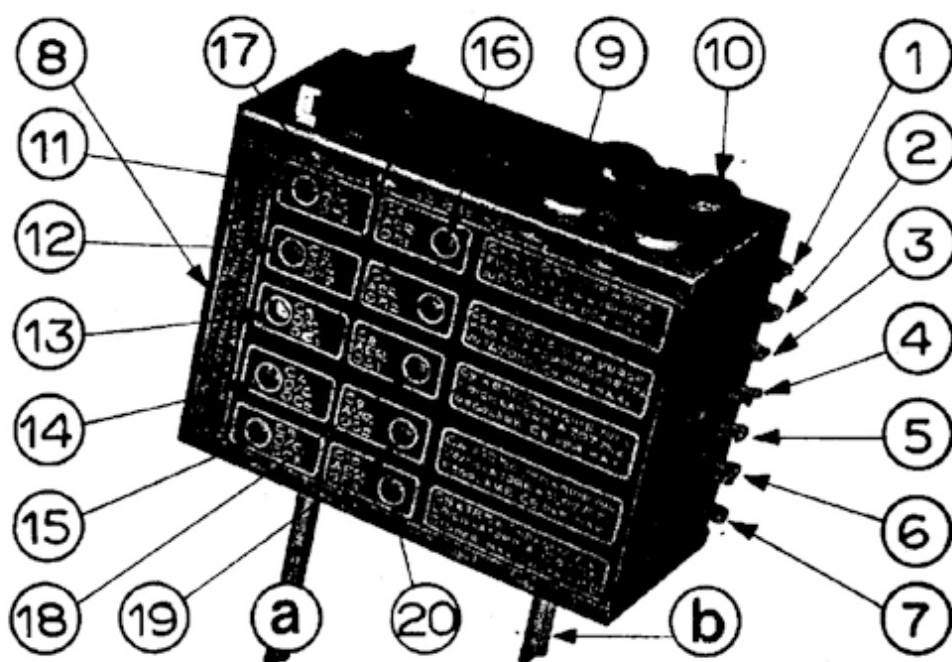
La disposizione dei compensatori del « P1 » Da 1 a 8, collegamenti già specificati nel testo; 9 padding OM1 (vite rossa); 10 padding OM2 (vite verde); 11 - 18 compensatori, dell'oscillatore e 19 - 20 compensatori antenna nella progressione OM1, OM2 OC1, OC2, OC3; a) commutatore di gamma a cinque posizioni più fono; b) comando della sintonia.
