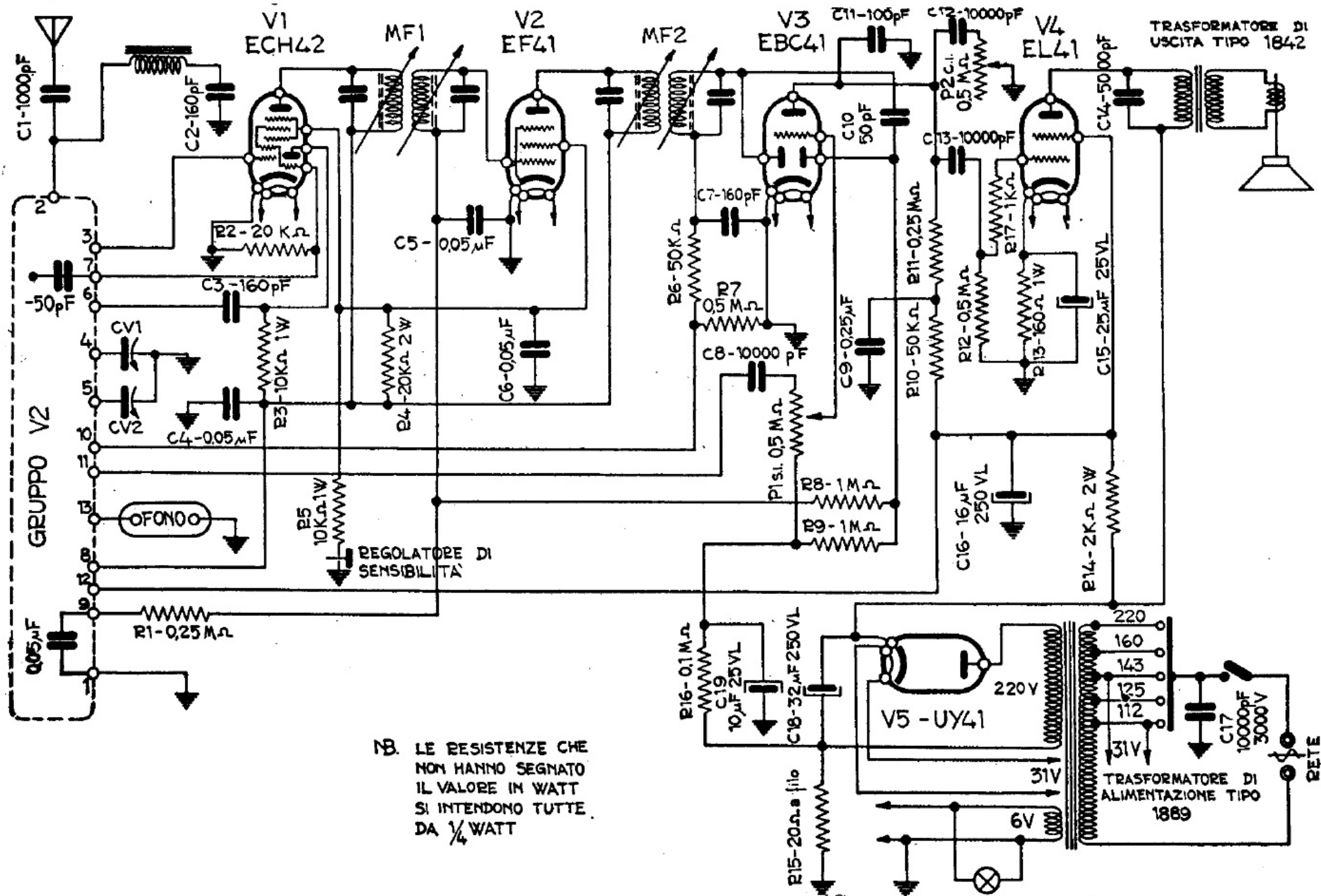
NOVA RADIO - Mod. R5 - Provvisto di gruppo alta frequenza mod. V2. Media frequenza 465 kc. Potenza d'uscita 4 watt indistorti.
