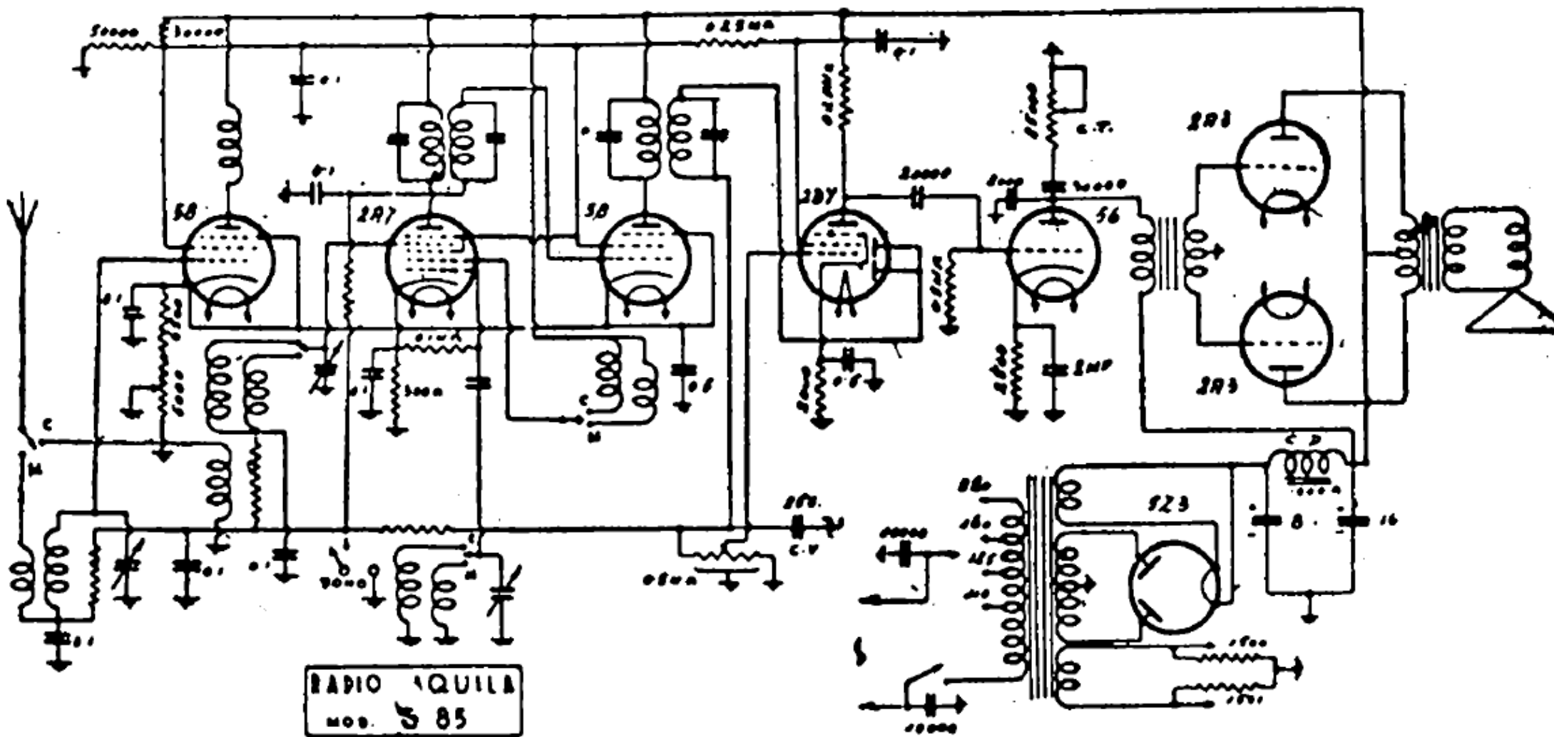
RADIO AQUILA — Mod. 8 85 — Produzione 1934. — Media frequenza 425 kc
