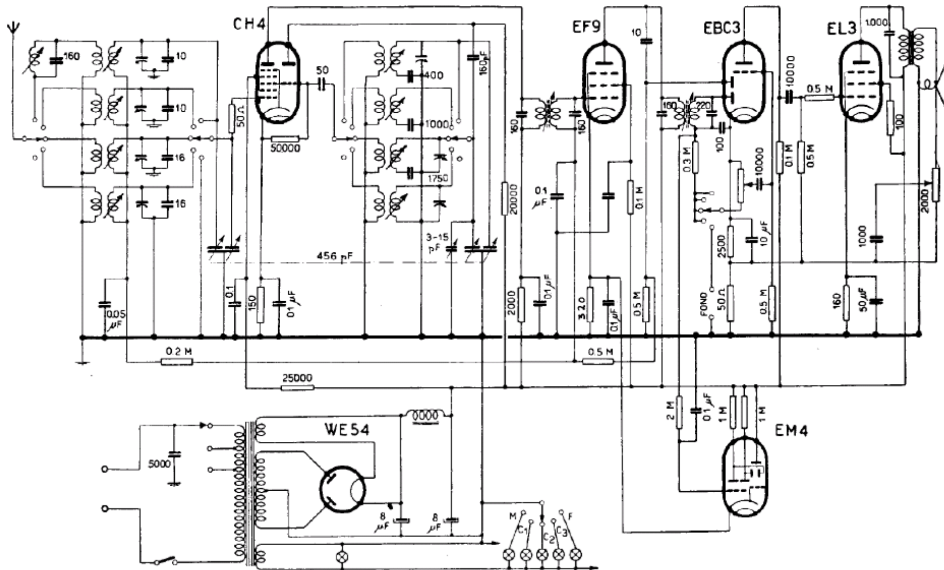
SUPERLA - Mod. 547 B - MF: 470 kc/s. ECH4 pl. 265, osc. 140, gr. 2,2. EF9 pL 265, sch. 100, gr. 2,4. EBC3 pl. 120, gr. 3,2. EL3 pl. 250, sch. 260, gr. 6,4. WE54 330 V p. Corr. tot. 67 mA. Prod. 1947-48.
