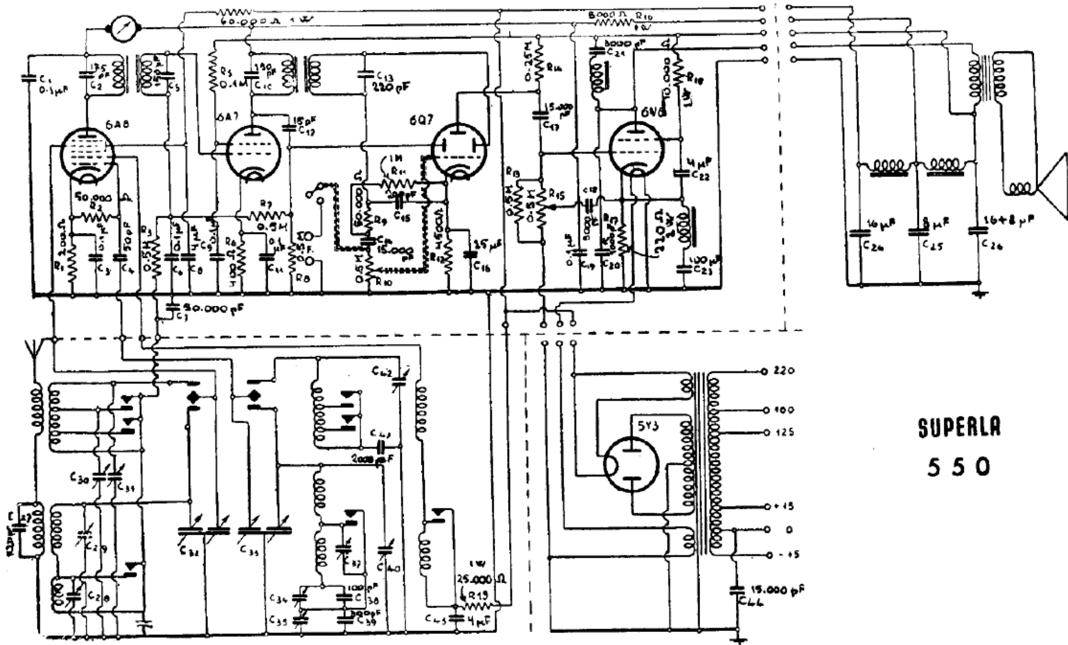
RADIO SUPERLA. — Mod. « 550 » e « 1550 » (prima e seconda serie). — Produzione 1939-1940. — Media frequenza: 468 kHz. — 5 \frac{1}{2} gamme d'onda. — Gamme d'onda: C1 (12,1-20,5 m.), C2 (18,7-32 m), C3 (30-51,2 m), m. (200-600), l. (700-2000 m.).
