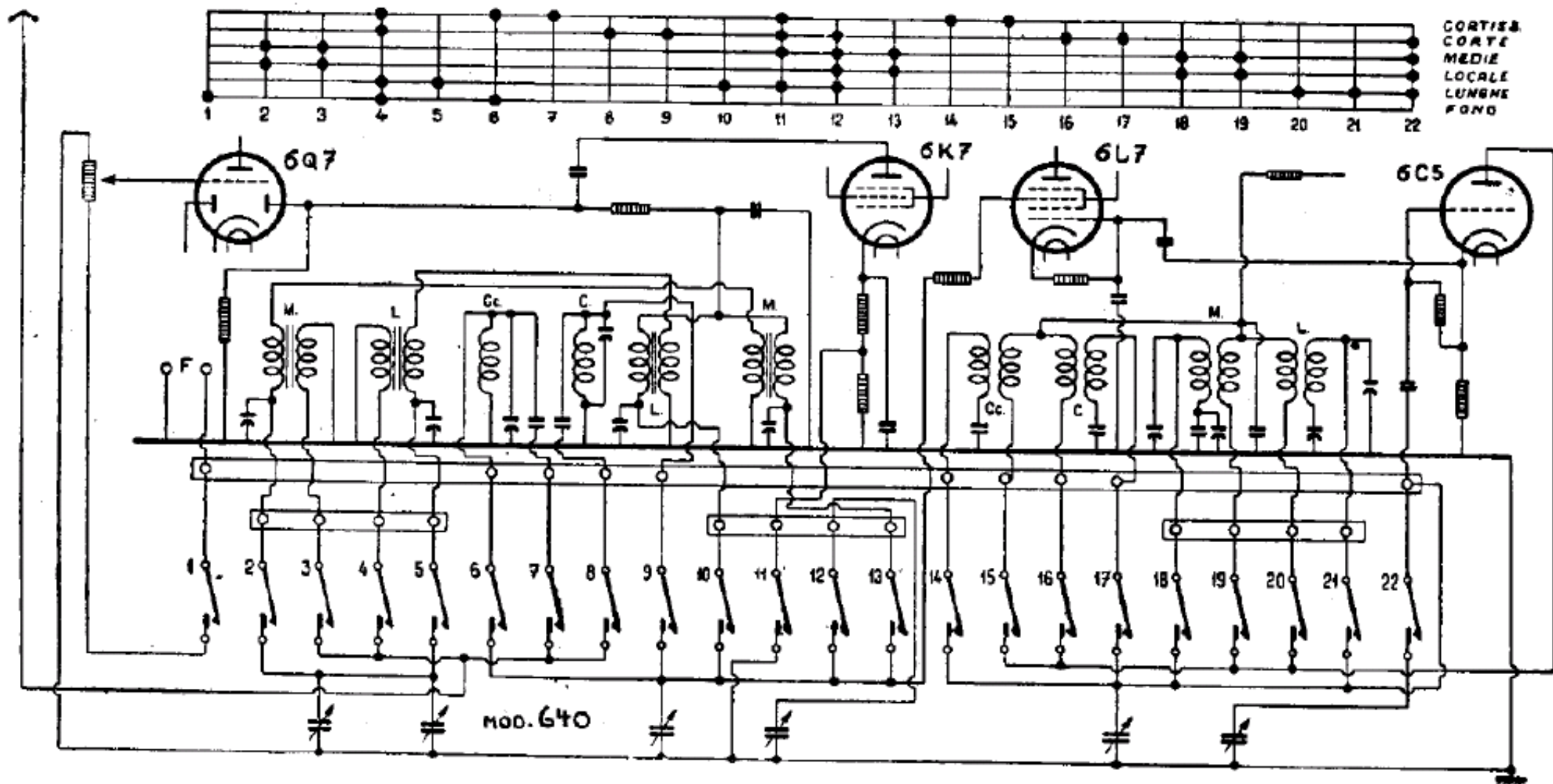
RADIO SUPERLA. — Mod. « 640 » e « 1640 ». - Particolari della tastiera per la ricerca automatica delle emittenti.
