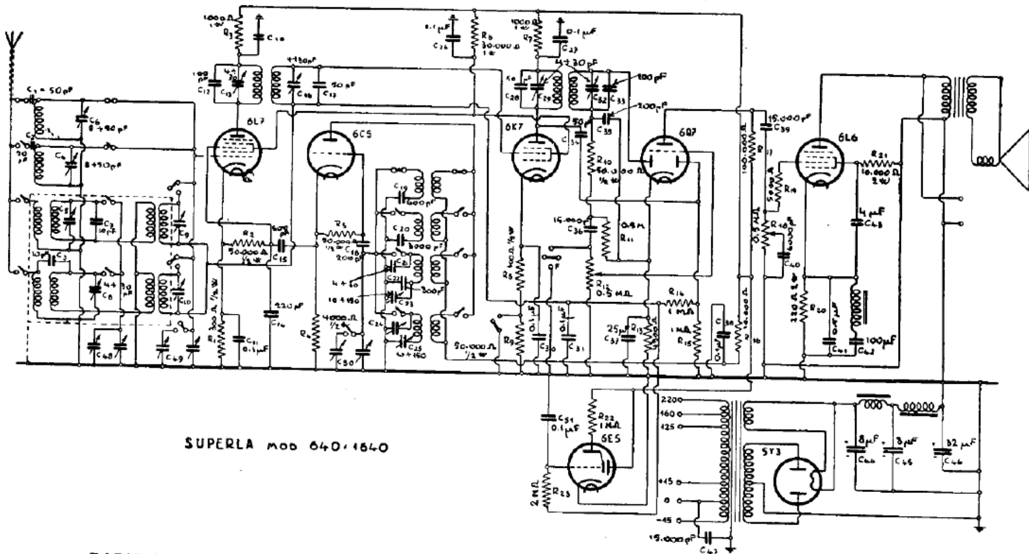
RADIO SUPERLA. — Mod. « 640 » e « 1640 ». — Produzione: 1939-1940. — Media frequenza: 468 kHz. — Gamme: c. c. (13,5-25 m), c. (19-50 m), m. (200-600 m), l. (700-2000 m). — Potenza d'uscita: ca. 4 watt.
