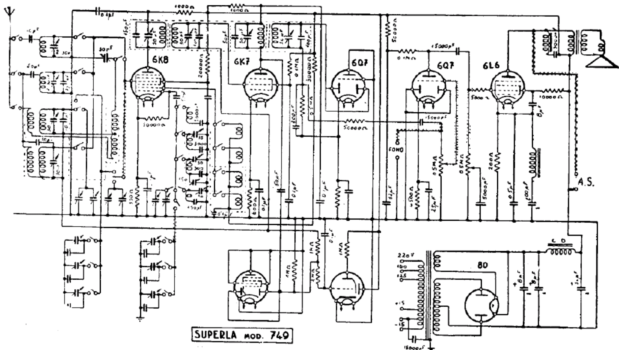
RADIO SUPERLA. — Mod. « 749 » e « 1749 ». Anche mod. « 740 » e « 1740 ». — Produzione 1938-39. — Gamme: cc. (13-70), c. (22-50), m. (200-600), l. (750-1950). — Media frequenza: 468 kHz.
