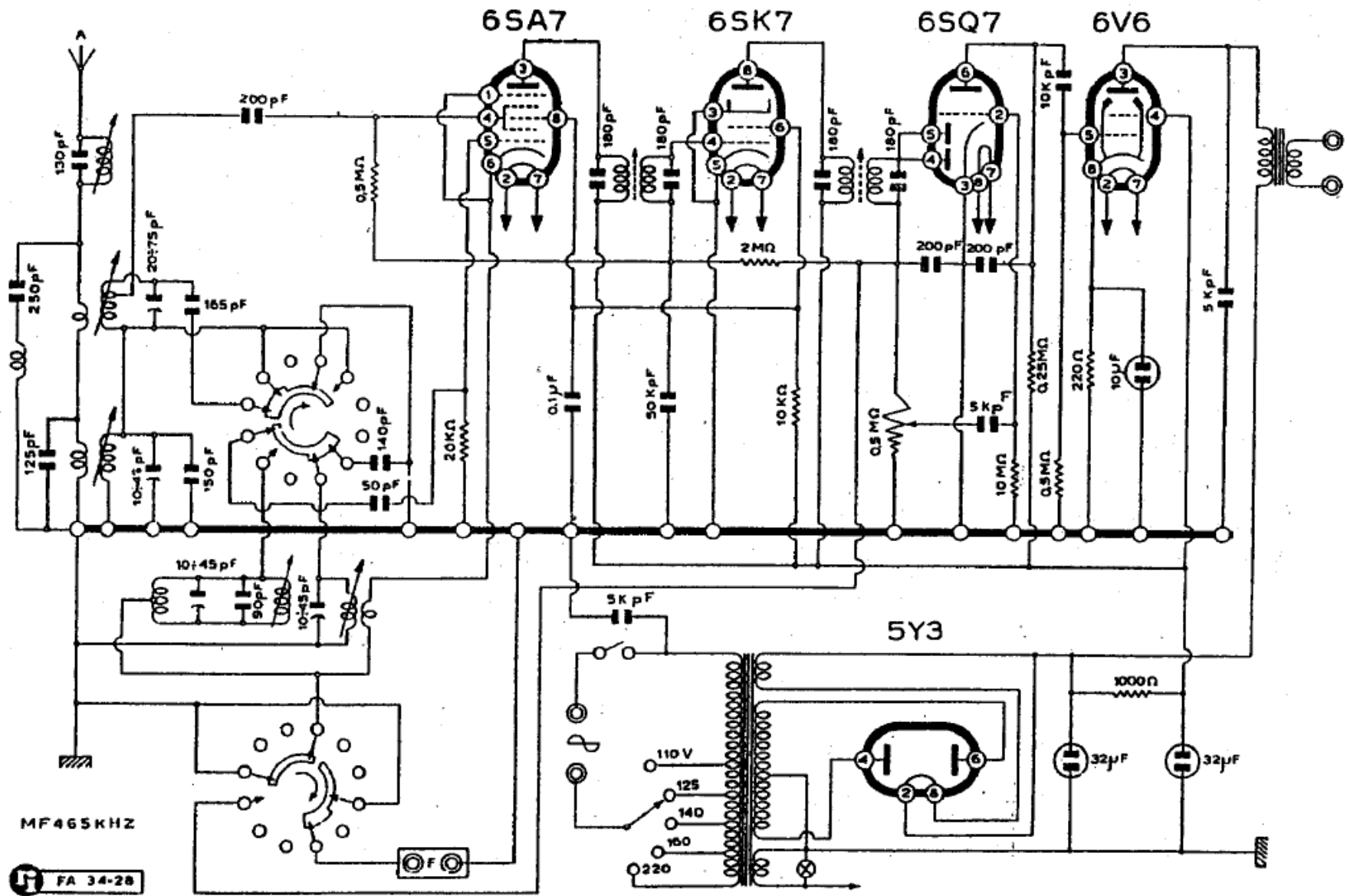
RADIO SUPERLA - Mod. Casa SP51
