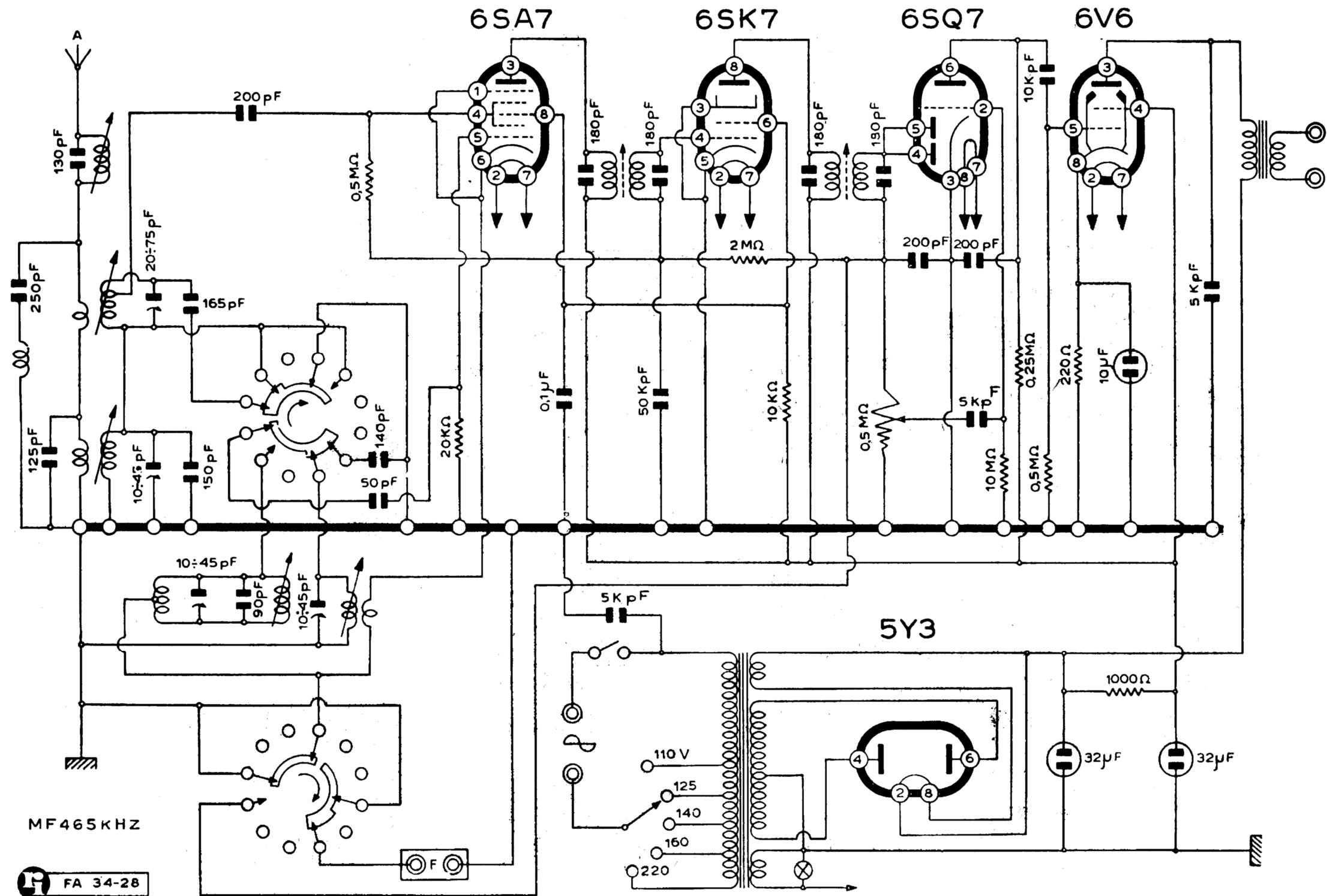
RADIO SUPERLA - Mod. Casa SP51
