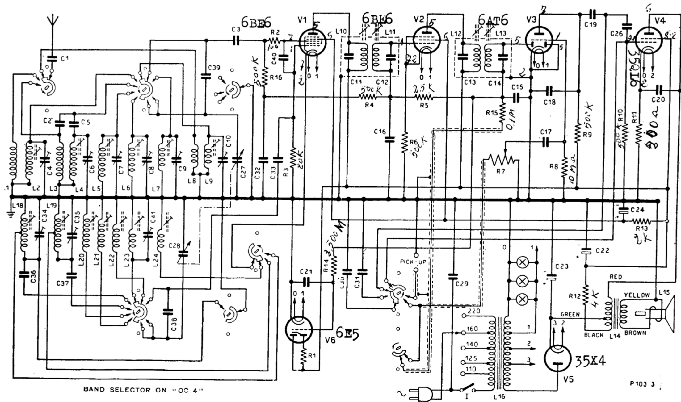
RADIO MARELLI - Mod. 137. Onde medie da 516 a 1615 kc/s; onde tropicali da 2170 a 5800 kc/s; banda OC1 da 5350 a 8500 kc/s; banda OC2 da 7850 a 11.800 kc/s; banda OC3 da 11.300 a 17.000 kc/s; banda OC4 da 16.900 a 27.150 kc/s. Media frecuencia a 455 kc/s.
