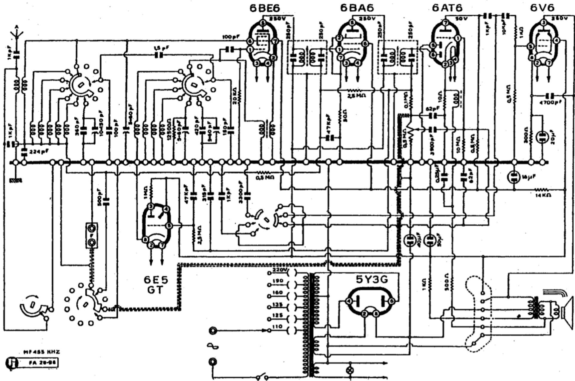
Radiomarelli 139
