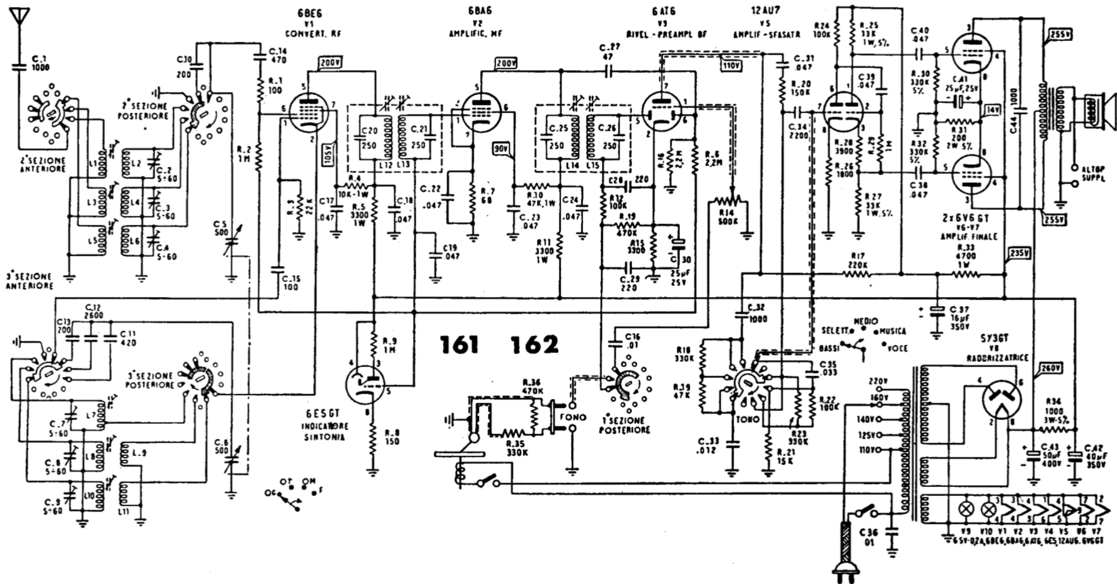
RADIO MARELLI - Mod. 161 e 162. Tre gamme, onde medie, tropicali e corte. MF a 455 kc/s. Impedenza altoparlante 8 ohm. Potenza d'uscita 7 watt. Consumo di corrente a 160 V = 0,54 A. Potenza assorbita 78 watt. Il mod. 161 è senza fonorivelatore.
