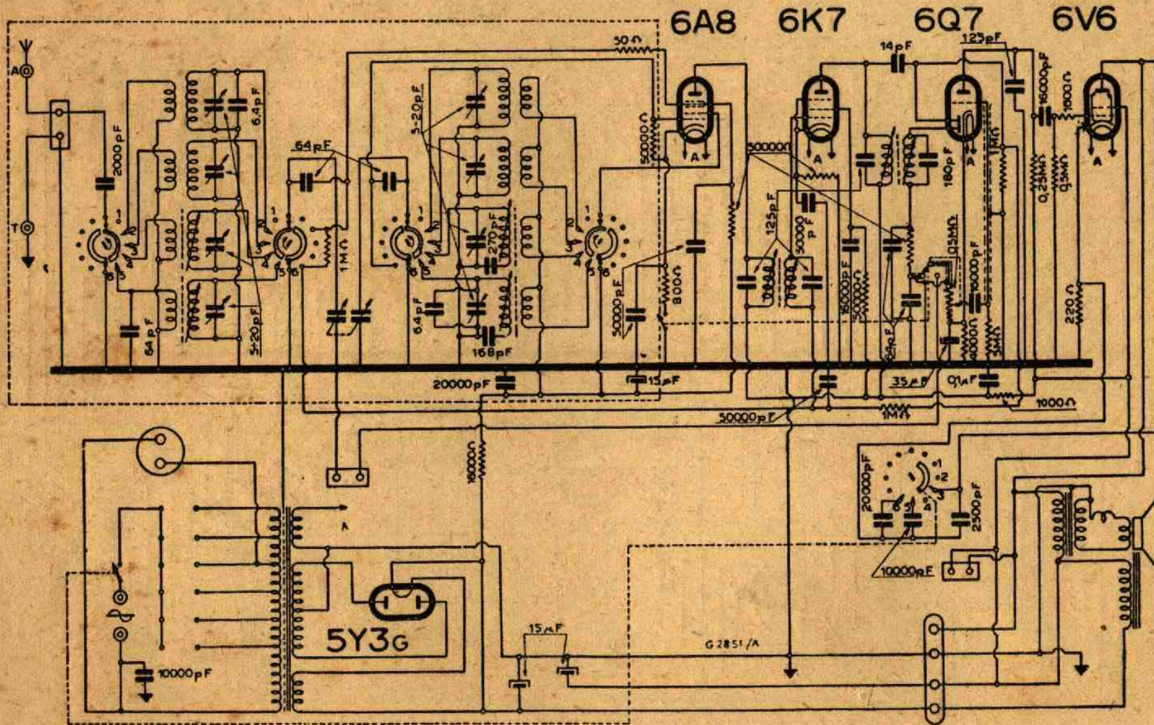
Mod. 8A05 Radioricevitore.
