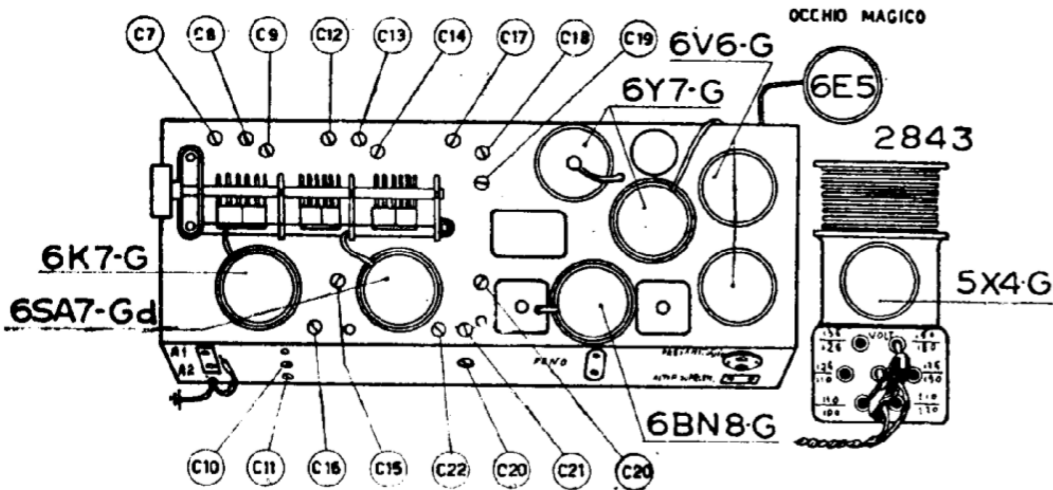
Il telaio del mod. « BA28 » con l'indicazione dei vari compensatori.
