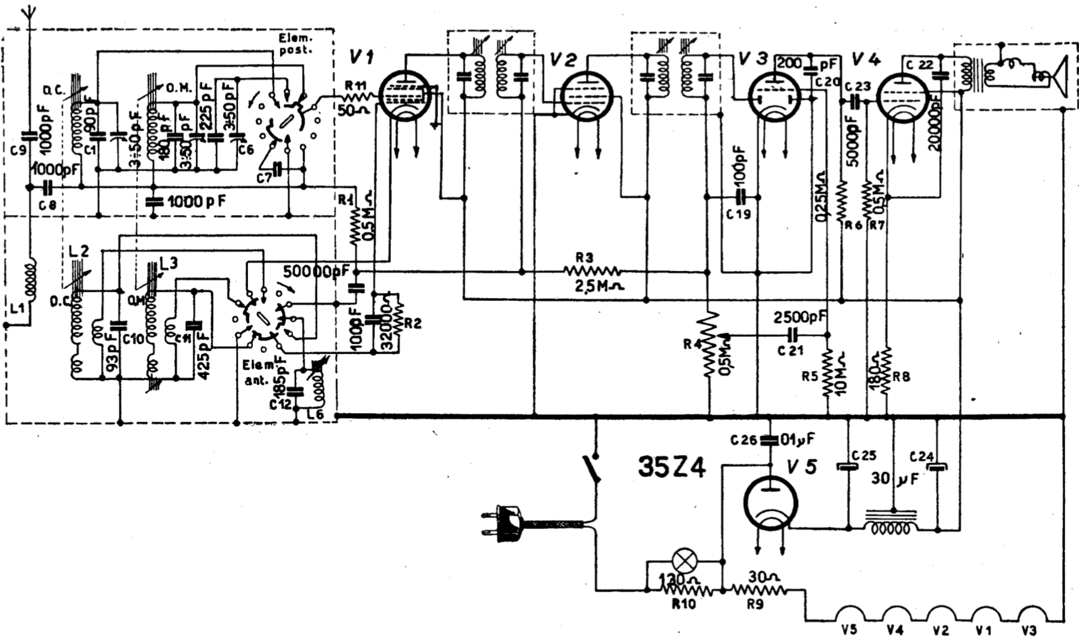
MARELLI 9U 65 - Serie Fido - Con sintonia a permeabilità. Onde medie e corte. Media frequenza: 470 kc/s. Produzione 1946. Per norme di taratura v. «Note di servizio».
