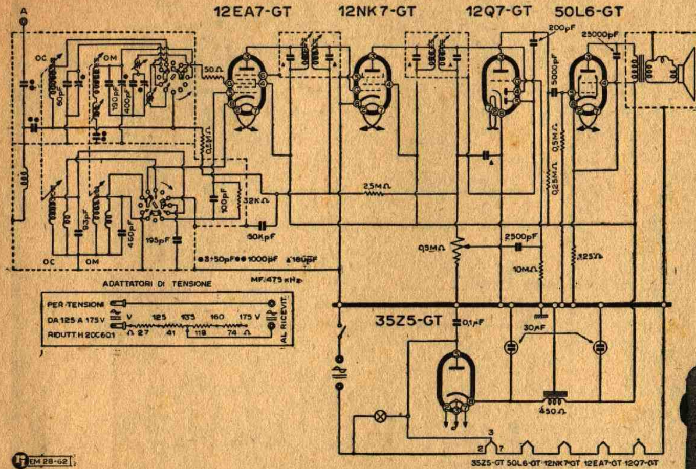
Lo schema elettrico del Radiomarelli mod. "9U65/c", e l'aspetto esterno dell'apparecchio.
