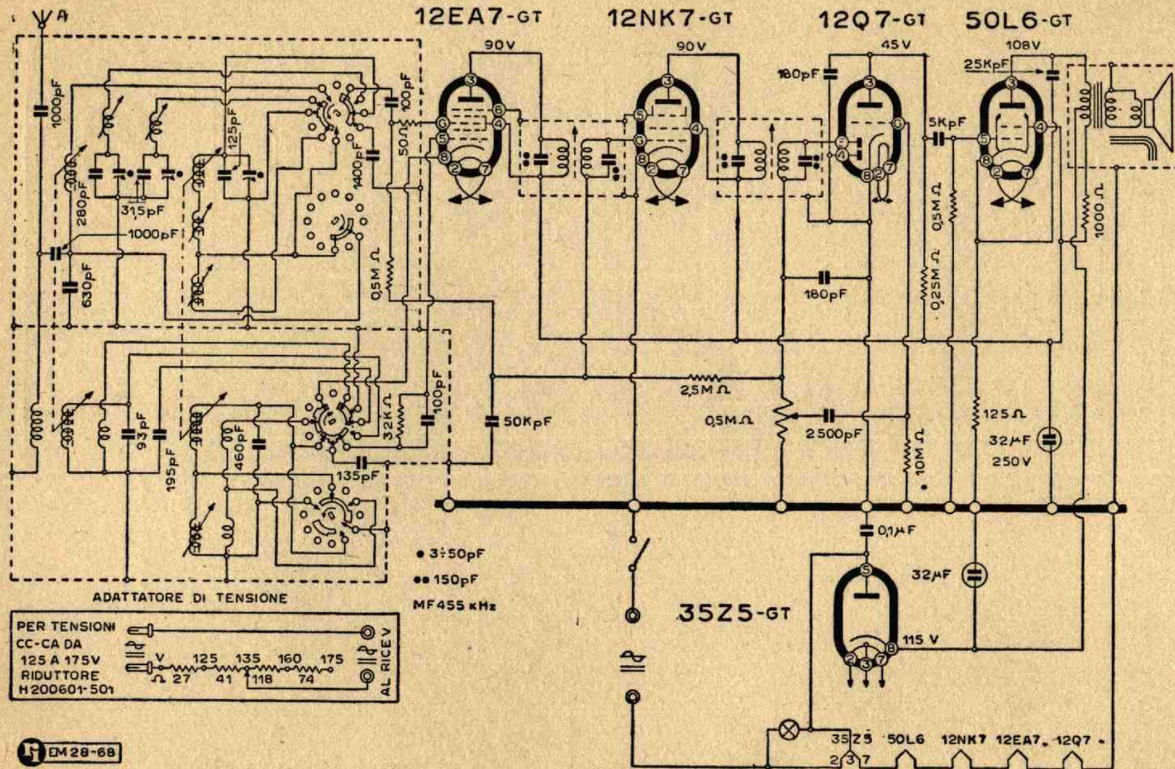
Lo schema elettrico del Mod. 9U65 G
