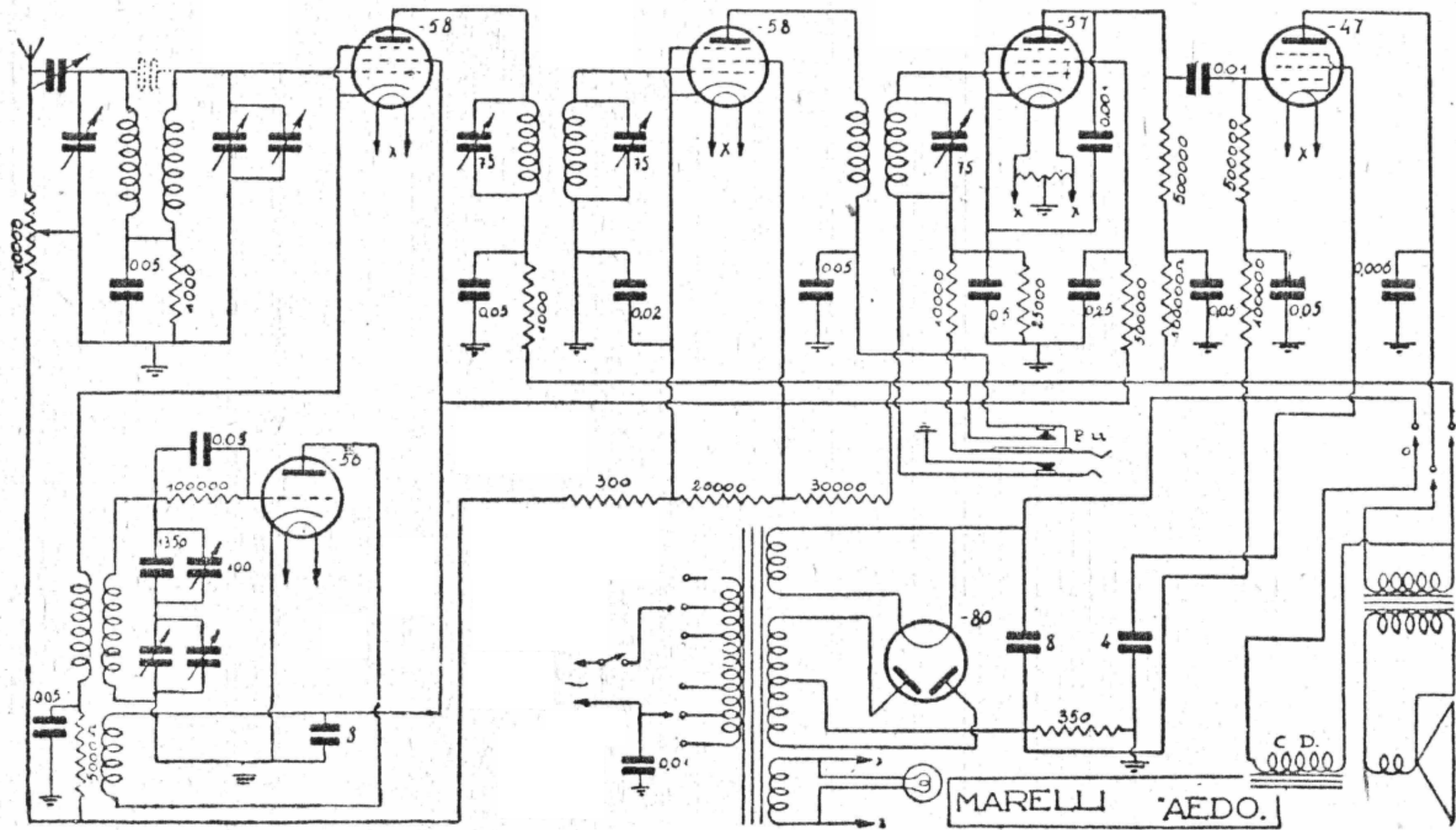
RADIO MARELLI. — Mod. Aedo. — Valvole e valori indicati nello schema. — MF: 175 kHz. — Prod. 1933-1934.
