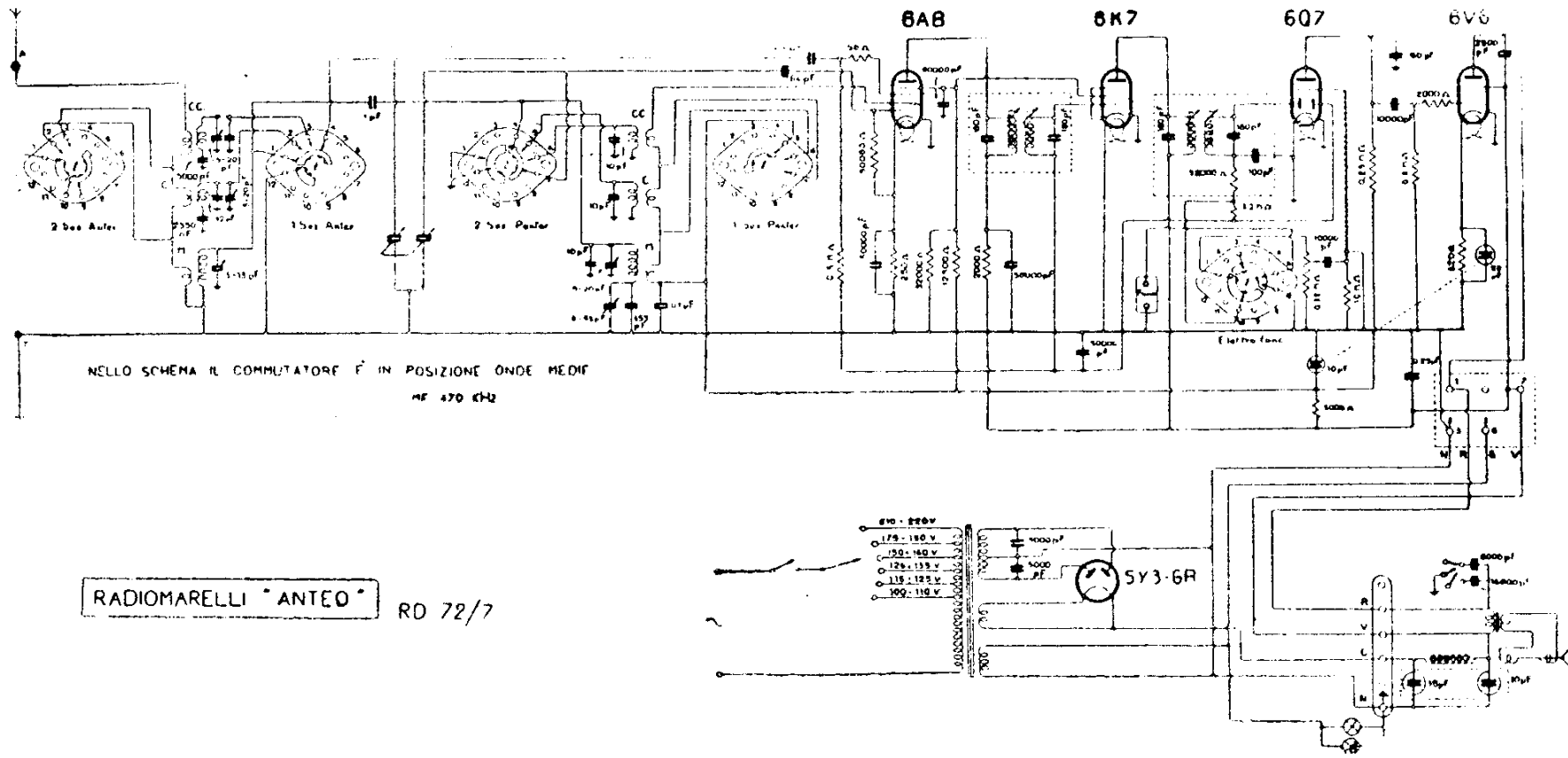
RADIOMARELLI - MOD. « ANTEO »
