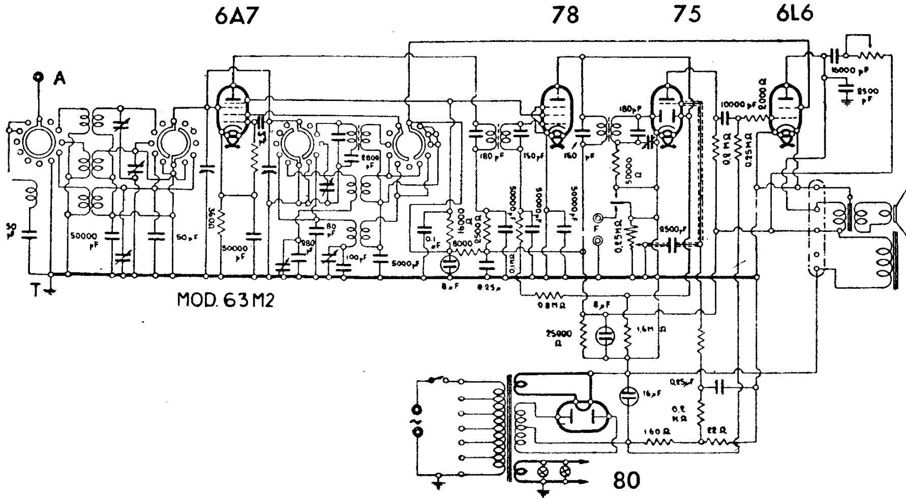
RADIOMARELLI - MOD. « AXUM »
