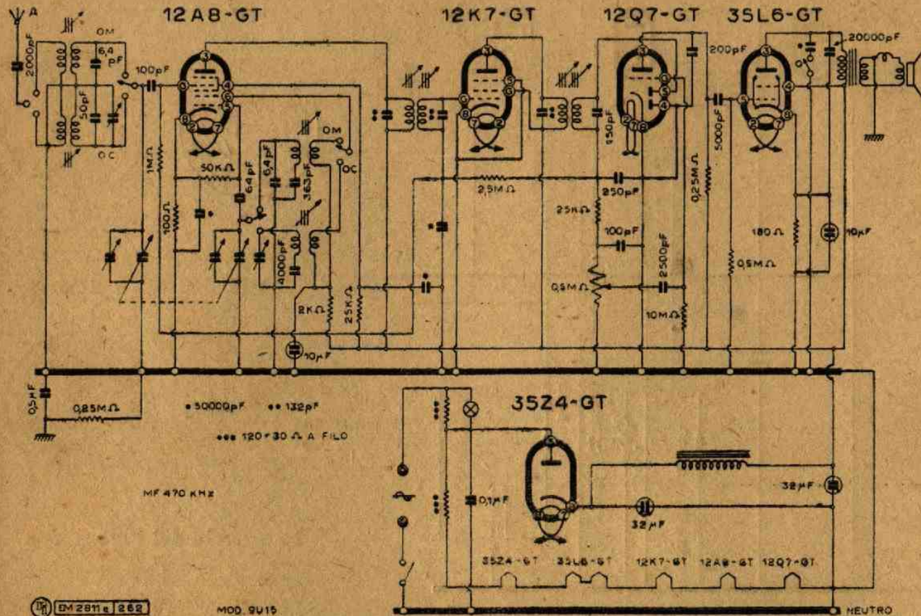
Lo schema elettrico 9U15 del Fido OC
