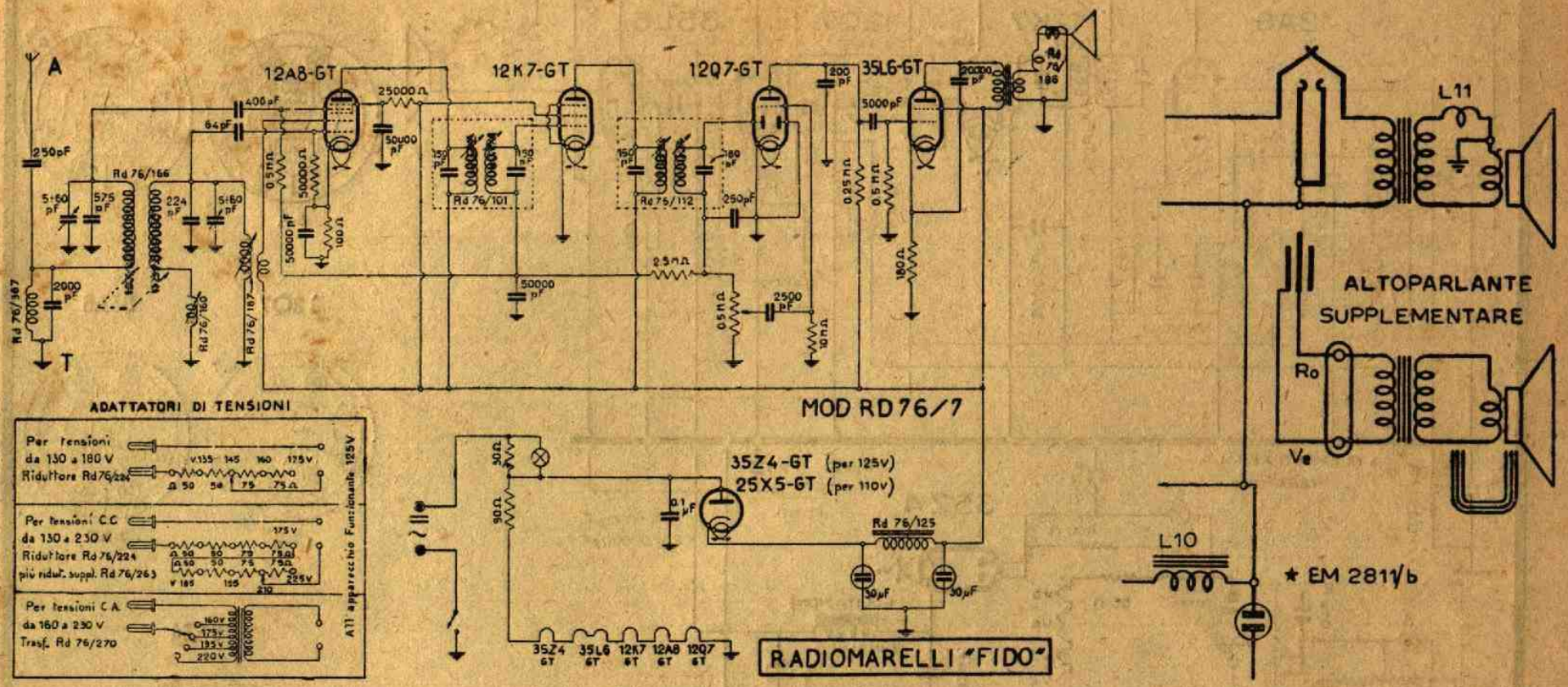
Lo schema del Fido E 3/0
