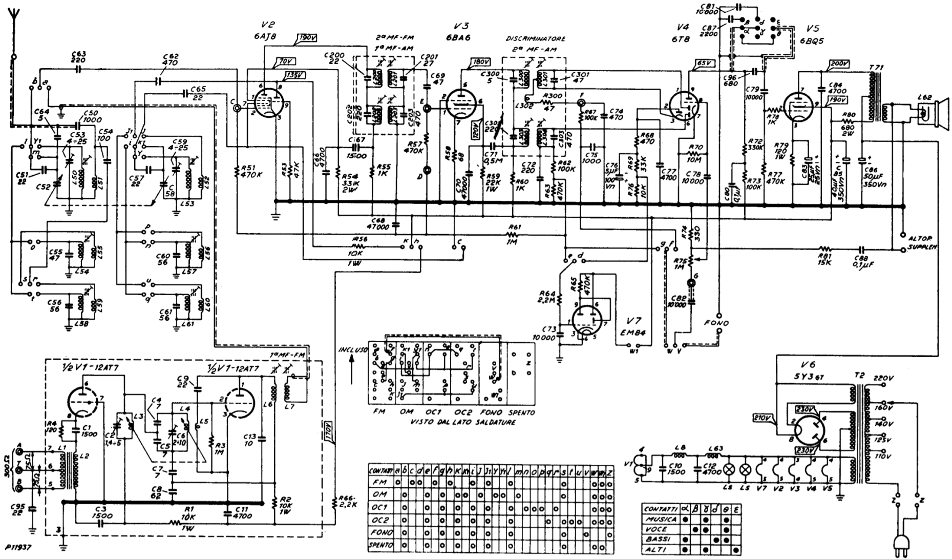
RADIO MARELLI - Mod. RD 196 e RD 198. Apparecchi AM/FM. Onde medie da 515 a 1640 kc/s; banda OC1 a 50 metri; banda OC2 a 25 metri; onde ultracorte (FM) da 87,5 a 100,5 Mc/s. Medie frequenze a 455 kc/s e a 10,7 Mc/s, Sintonia AM con condensatore variabile; sintonia FM a permeabilità variabile. Potenza d'uscita con 10 per cento di distorsione: 2,5 watt. Potenza assorbita: 50 watt. (Posizione condensatori e induttanze da regolare, e funicella scale, come modd. 171 e 176, v. tavola).
