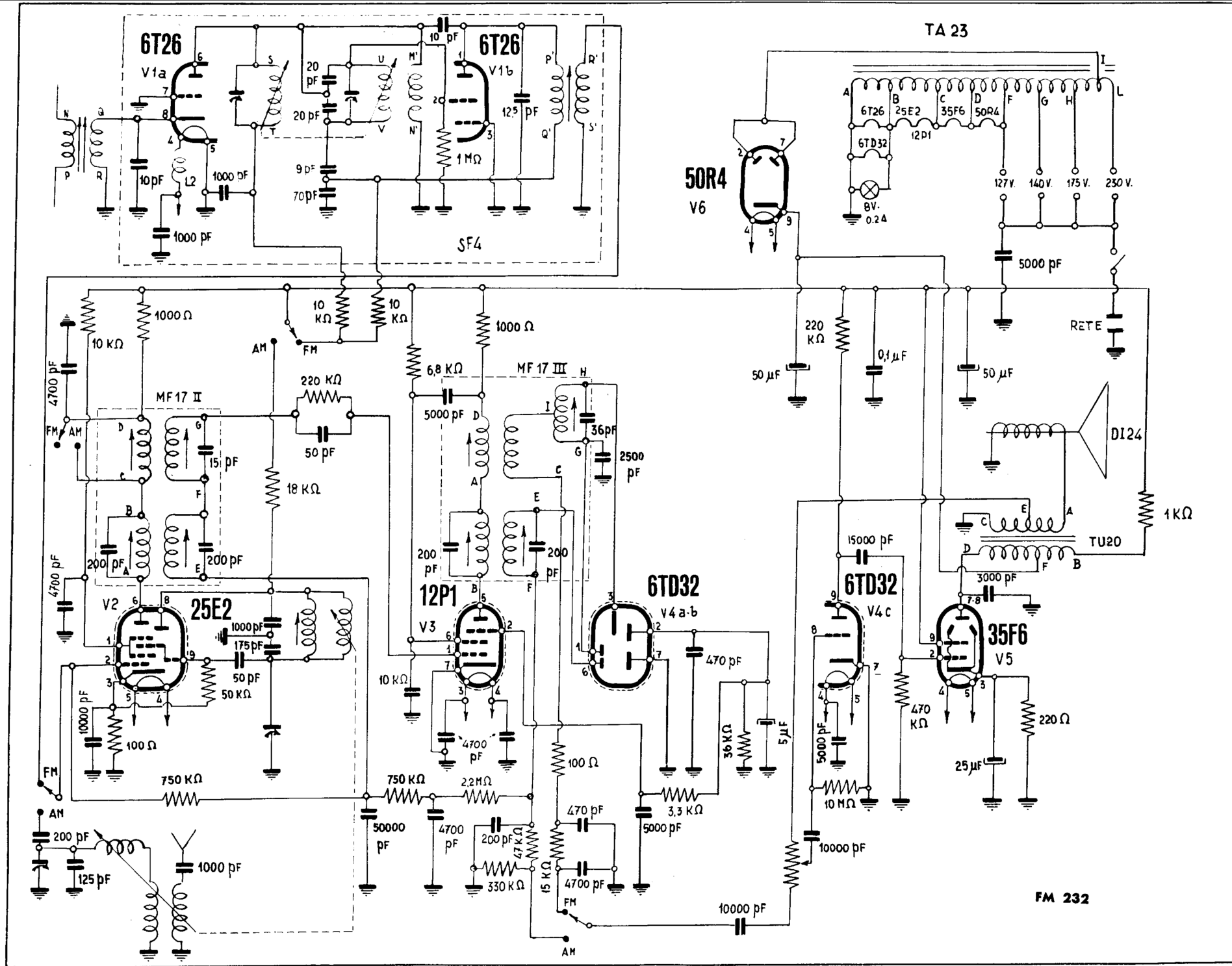
RAYMOND (GARUFI) - Mod. FM 232. Apparecchio AM/FM della serie Anie. Una gamma onde medie da 520 a 1620 kc/s e una banda ad onde ultracorte FM da 88 a 101 Mc/s. Media frequenza AM a 471 kc/s, media frequenza FM a 10,7 Mc/s. Potenza d'uscita 3 watt. Assorbimento 45 watt.
