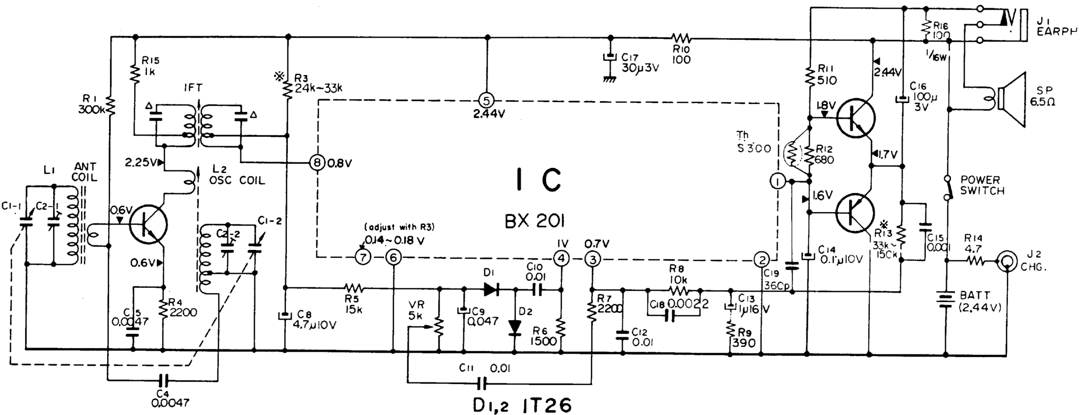
Fig. 8.22. - Schema dell'apparecchio Sony ICR-120.
