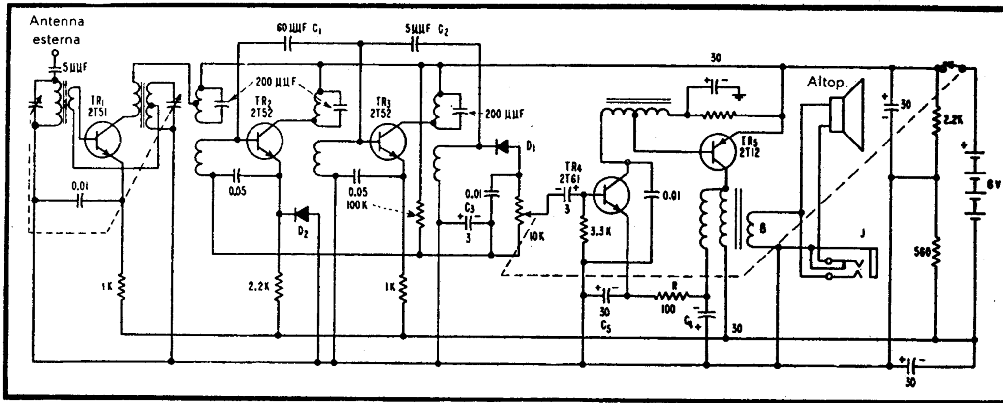
SCHEMA ELETTRICO DEL RADIORICEVITORE « SONY TR-55 » DELLA TOKYO TSUSHIN KOGYO, Ltd.
