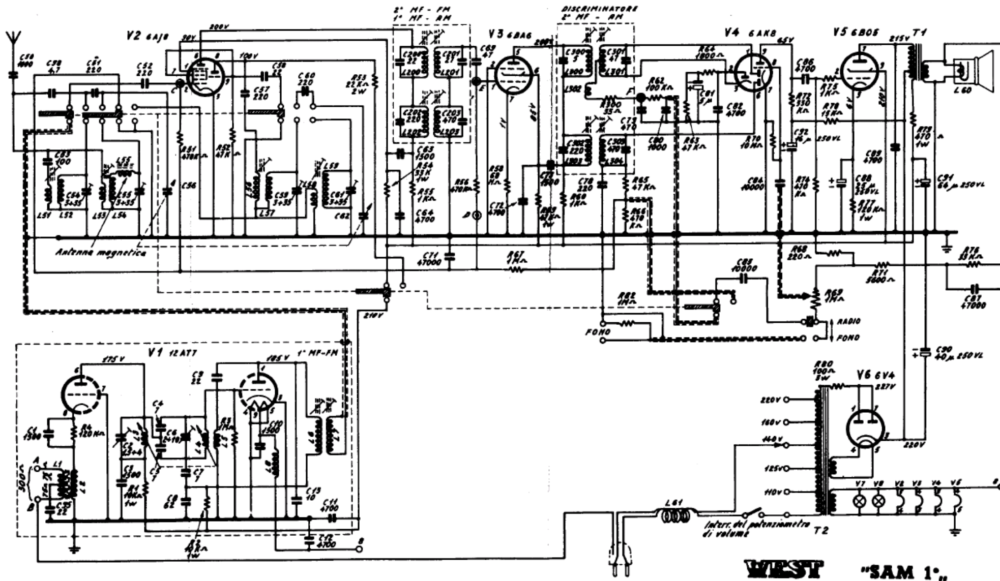
WEST RADIO-TV - Mod. SAM 1°. Apparecchio AM/FM con una gamma onde medie, una banda onde corte e una banda onde ultracorte. Media frequenza AM a 455 kc/s, media frequenza FM a 10,7 Mc/s. Resa d'uscita 2,5 watt. Consumo 42 watt.
