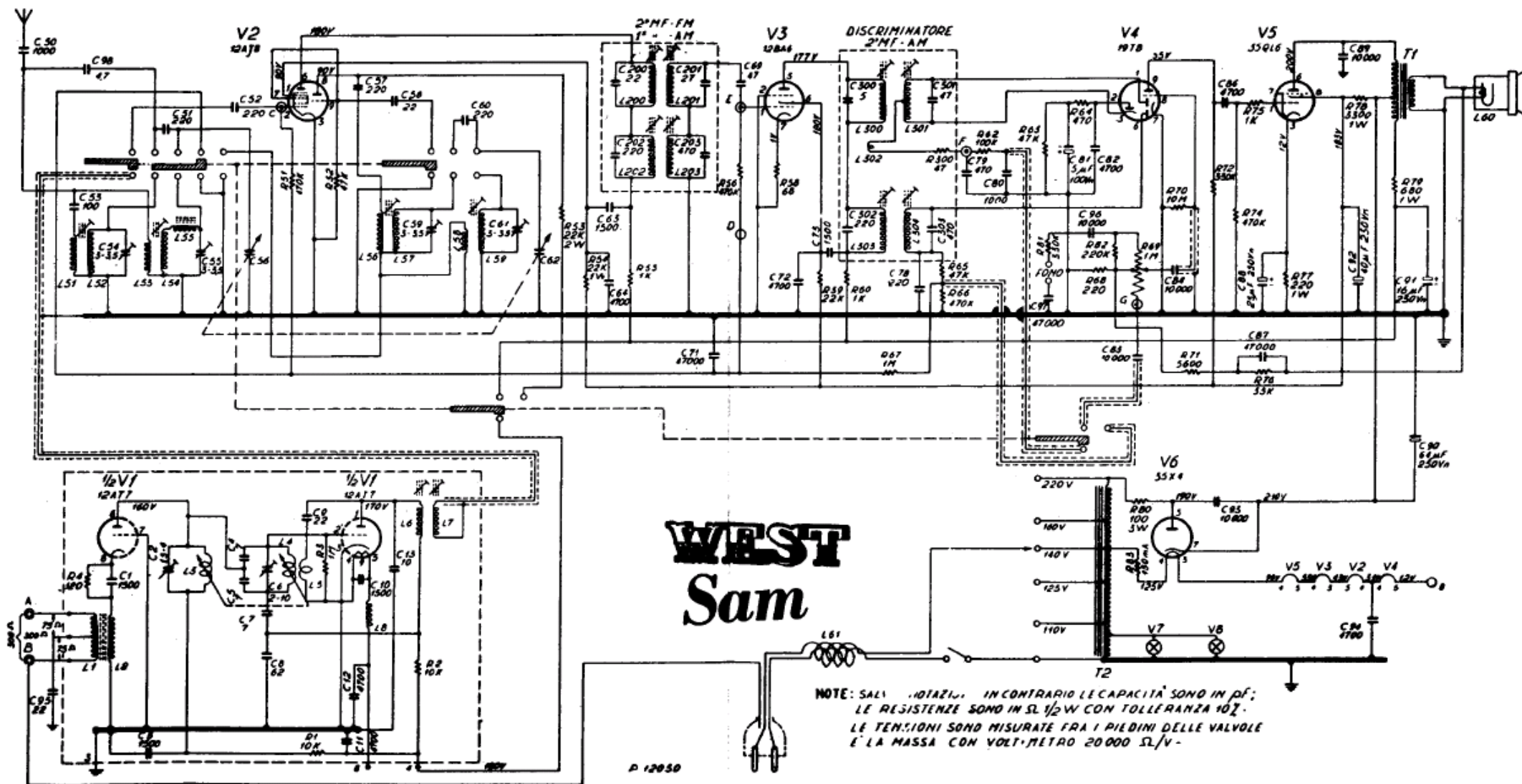
WEST RADIO-TV. Apparecchio AM/FM, con una gamma onde medie, una banda onde corte e una banda onde ultracorte. Media frequenza AM a 455 kc/s, media frequenza FM a 10,7 Mc/s. Potenza d'uscita 2,5 watt. Consumo 40 watt.
