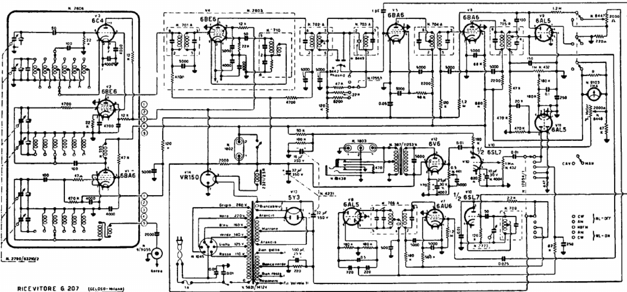
GELOSO - Mod. professionale per onde corte G 207 - R.
