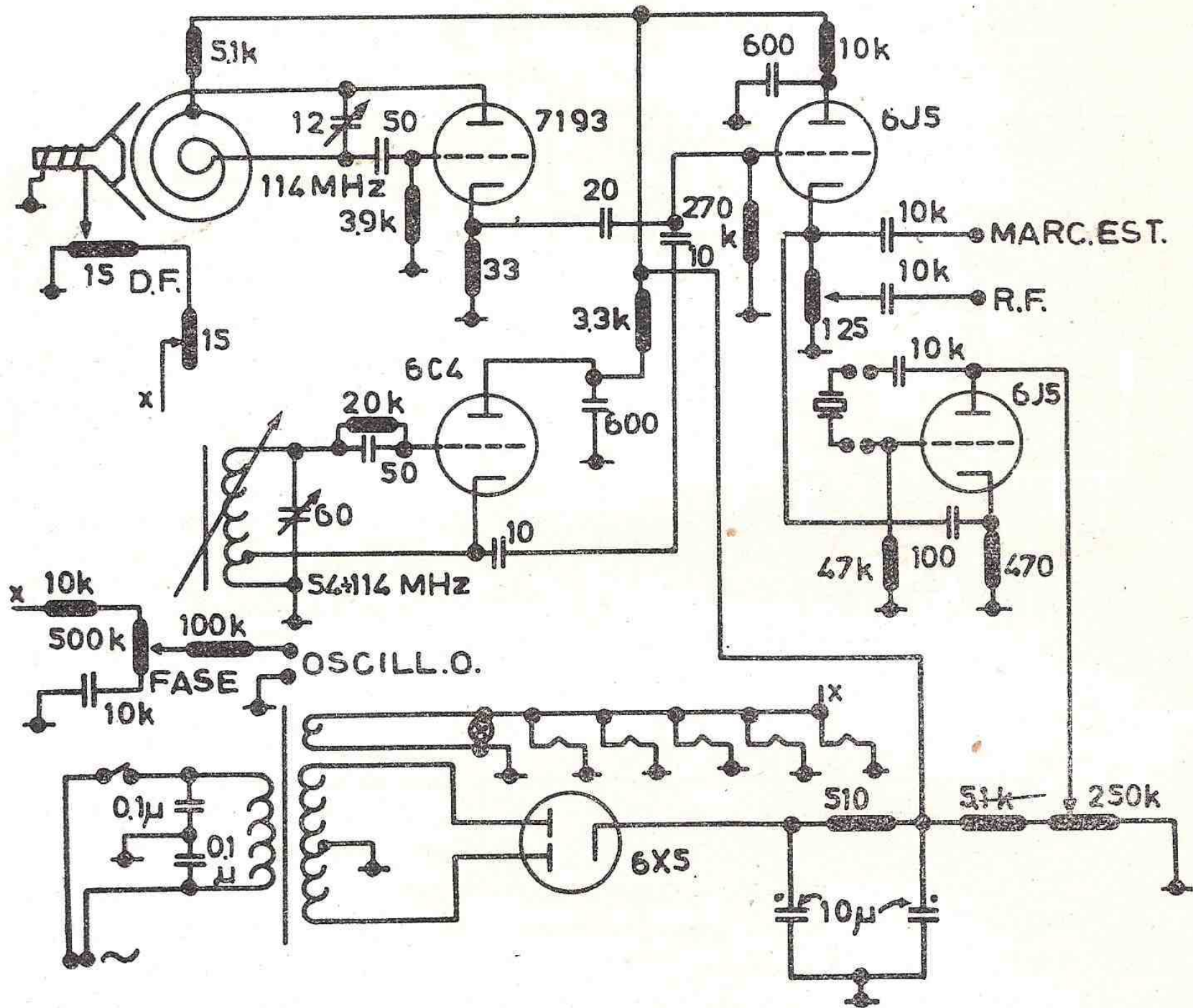
Fig. 76. - Vobulatore e marcatore Eico 360.
